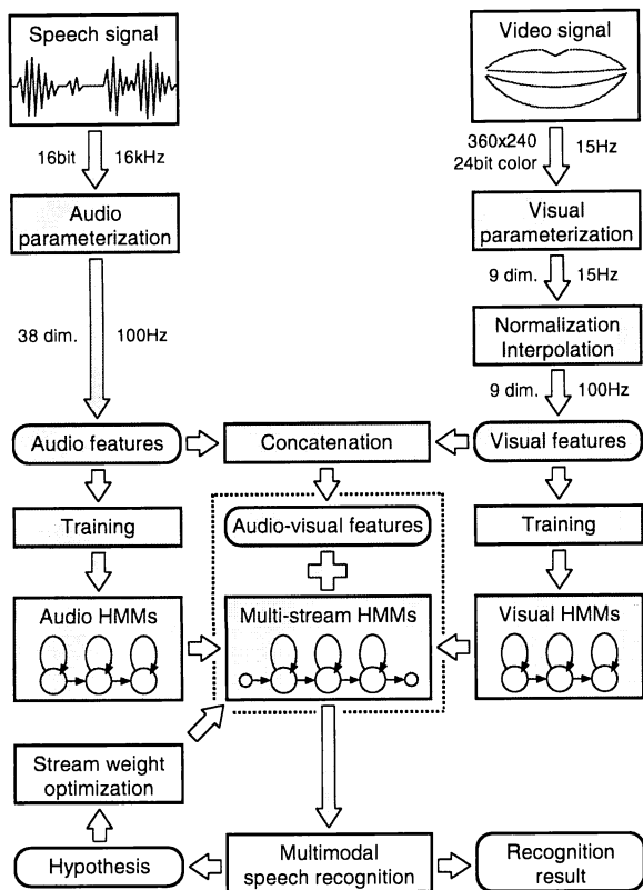
図 1: マルチモーダル音声認識システム
