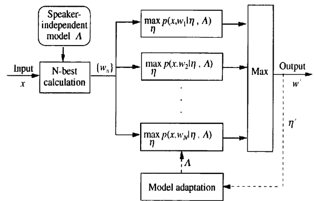
図 2 N-best 仮説に基づく話者適応化法を含む音声認識システムの構成
