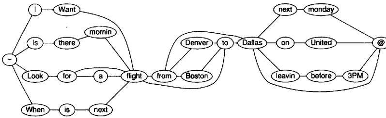
図3 ECGIアルゴリズムで生成される文法ネットワークの例 Fig. 3 An example of a network derived by ECGI algorithm.
