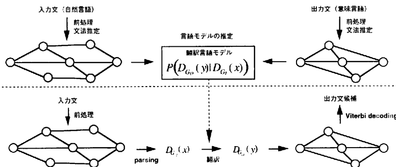
図2 統計的言語モデルによる音声理解の言語処理 Fig. 2 Language processing for speech understanding using a stochastic language model.
