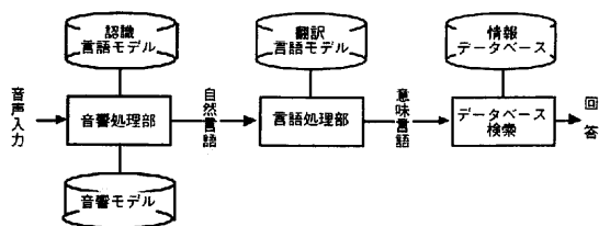
図1 音声理解システムの一構成例
