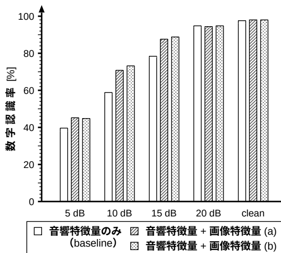
図 3: 認識結果
