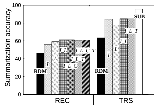
図 3. 要約率 80% 時における要約正解精度
