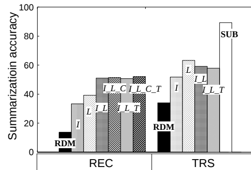
図 2. 要約率 50% 時における要約正解精度
