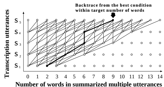
図 1. 複数発話の音声要約のための動的計画法の計算領域の例
