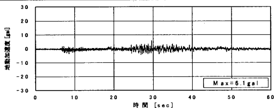
(a) 地動加速度：東西方向
