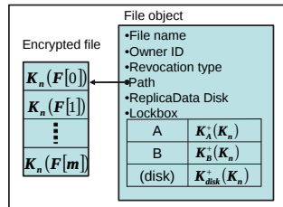
図3 データ構造
