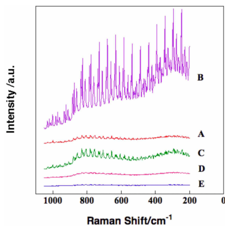
図2 テラス構造を有する被覆微小球の励起実験
