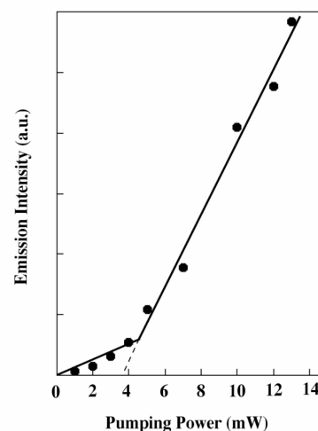
図3 励起強度依存性
