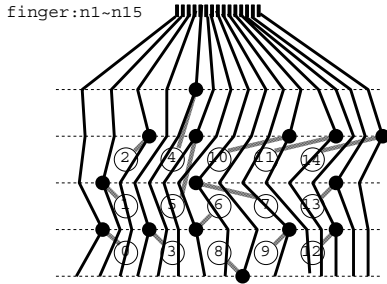
図 12: ビア配置最適化後の配線経路
