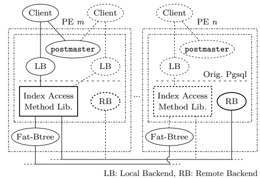
図2 PE内の構成 Fig. 2 A structure of a PE
