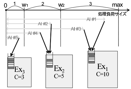
図 3 OXTHAS-N スケジューリングの例 ( N = 3 ) Fig. 3 An example of OXTHAS-N scheduling. ( N = 3 )
