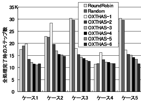
図 5 エグゼキュータの性能差の違いによる総処理ステップ数
