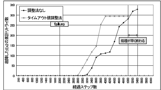
図 9 タイムアウト値調整法の有無による OXTHAS の故障したエグゼキュータ 2 の累計リトライ数の変化
