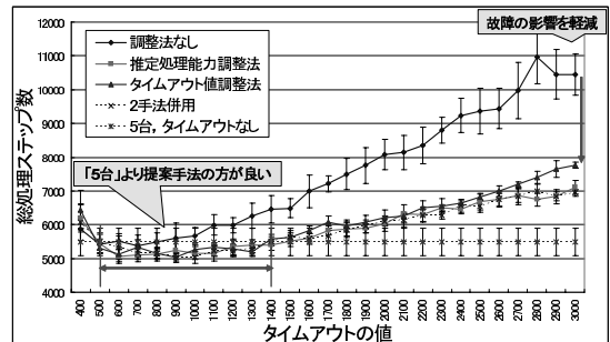
図 7 故障時における再割当手法の違いによる総処理ステップ数の比較
