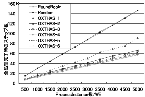
図 6 各プロセスインスタンス数における総処理ステップ数
