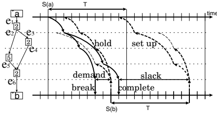
図 5: 遅延余裕量 \text{slack} と遅延要求量 \text{demand} .
