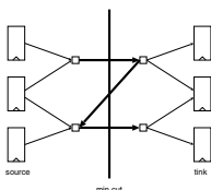
図 10: 1つのパス上の枝が最小カットに 2 以上含まれる例。有向枝の容量は全て 1。
