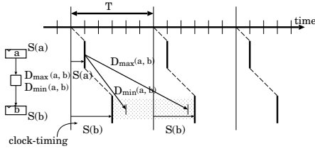
図 2: 同期回路のタイミング制約.
