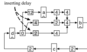
図 3: 回路 G に遅延を挿入した回路 G' .
