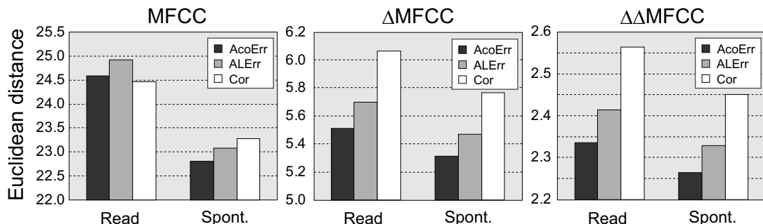
Fig. 2 音響的誤りフレーム，音響・言語的誤りフレーム，正解フレームにおける原点からの距離の違い
