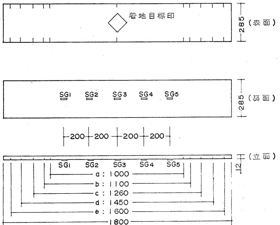
図-3・3 模擬床の詳細
