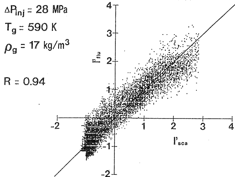
図 3 - 8 散乱光強度分布と蛍光強度分布の相関図
