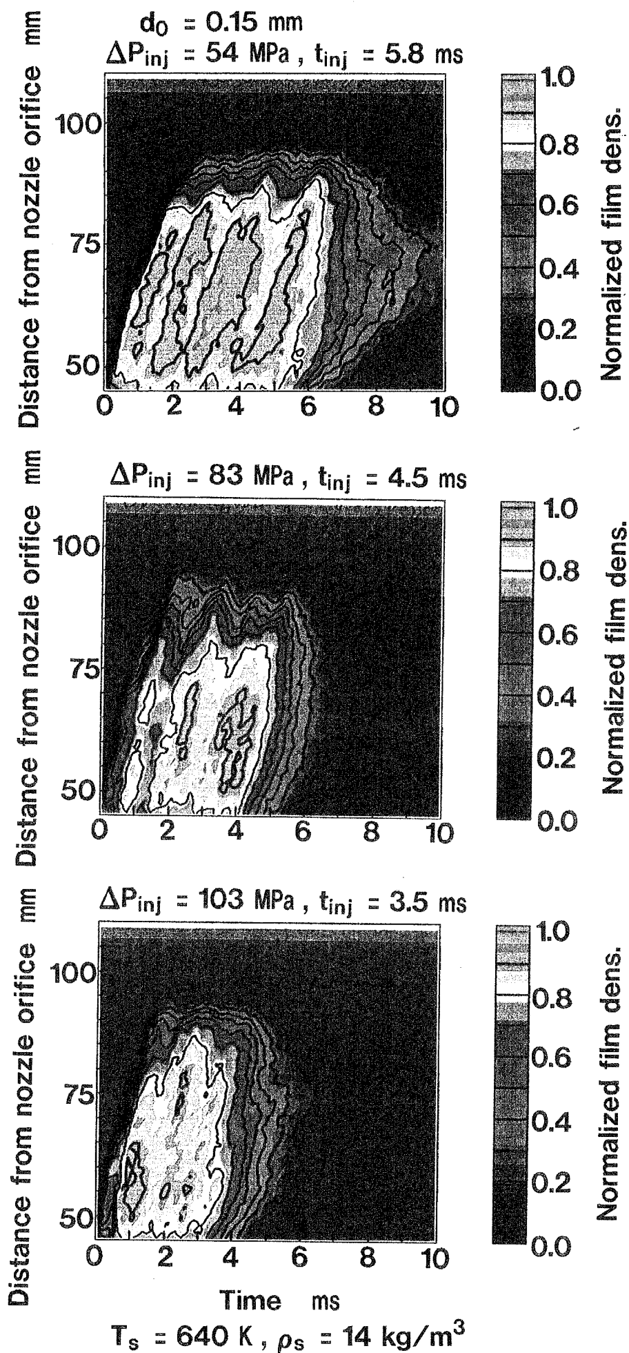
図 3-21 蒸気可視化画像の噴霧中心軸上のフィルム濃度分布の時間変化
