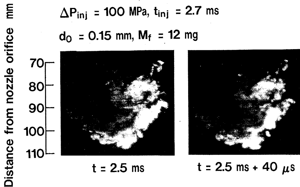
図 B - 1 40 \mu\text{s} の時間差で撮影された同一噴霧火炎内のすすの散乱光画像
