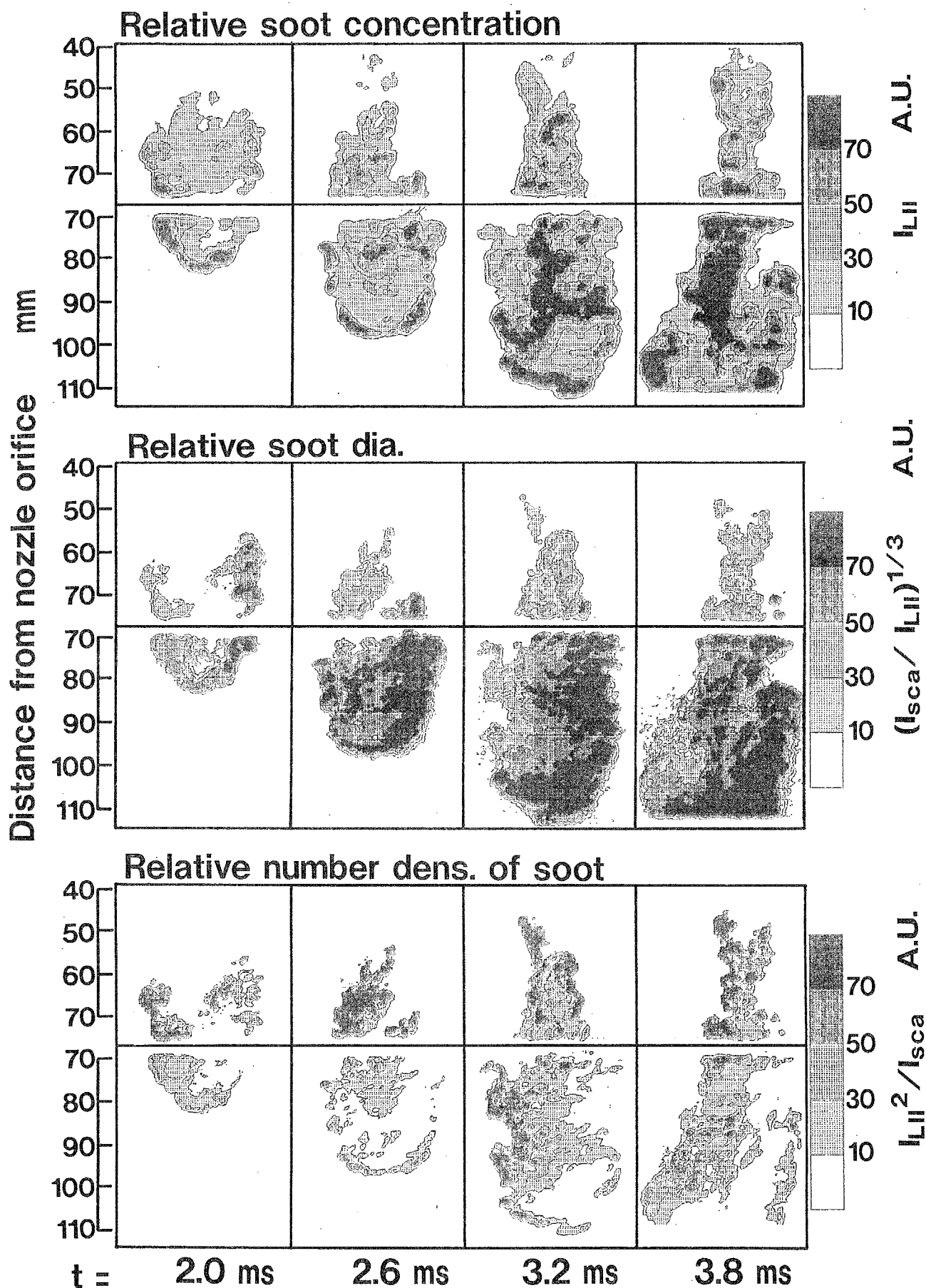
図 4 - 7 火炎断面内相対すす濃度分布 (上段)
