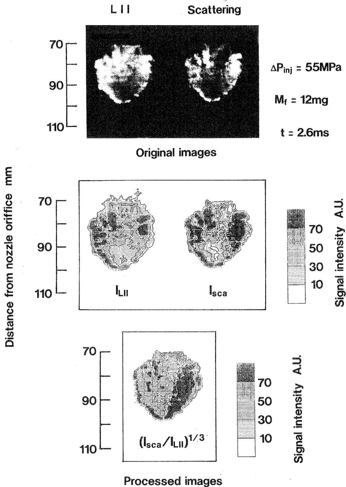
図 4 - 4 レーザシート光上の赤熱すす粒子群からの 輻射光画像と散乱光画像の例（上段） LII 光強度（中段左）と LIS 光強度（中段右） 相対すす粒径分布（下段）
