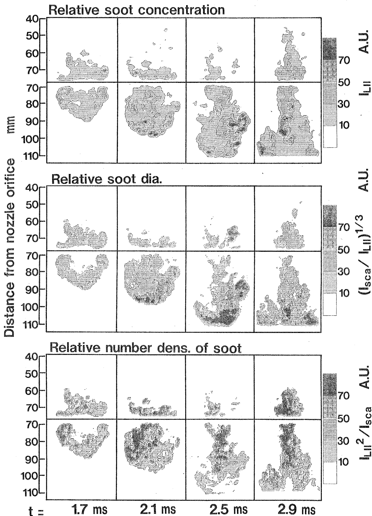
図 4 - 8 火炎断面内相対すす濃度分布 (上段)
