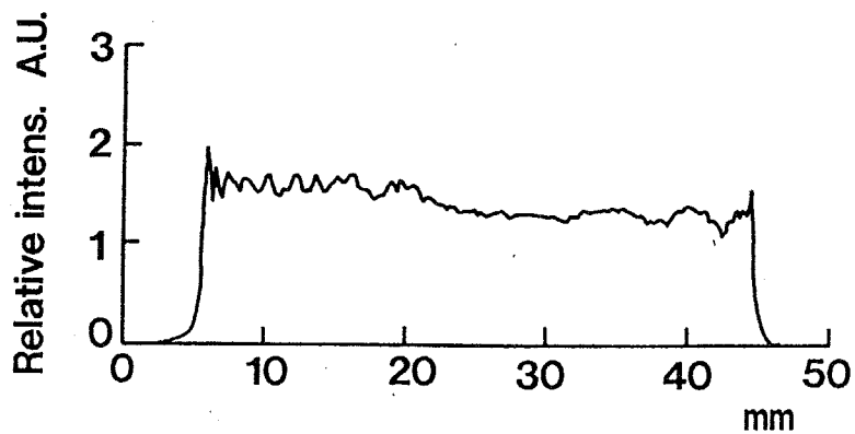
図C-3 シート光のエネルギー分布 (YAGレーザーの場合)
