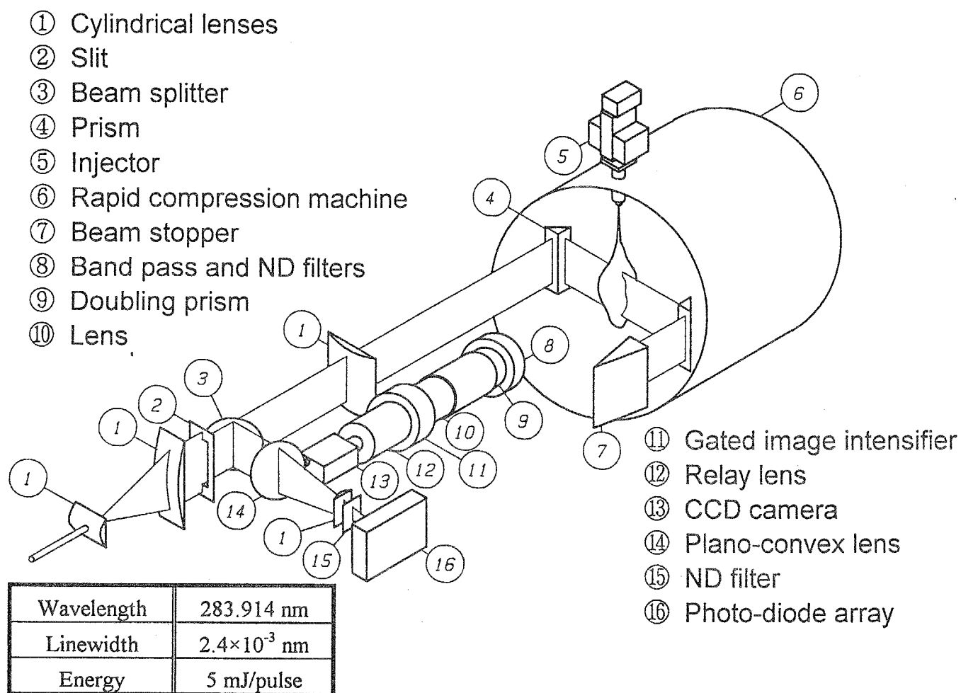
図 6 - 1 火炎内すすとOHの同時2次元可視化のための撮影光学系
