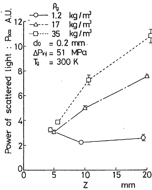
図 2 - 1 6 雰囲気気密度が噴霧断面内燃料からの散乱光パワーに及ぼす影響
