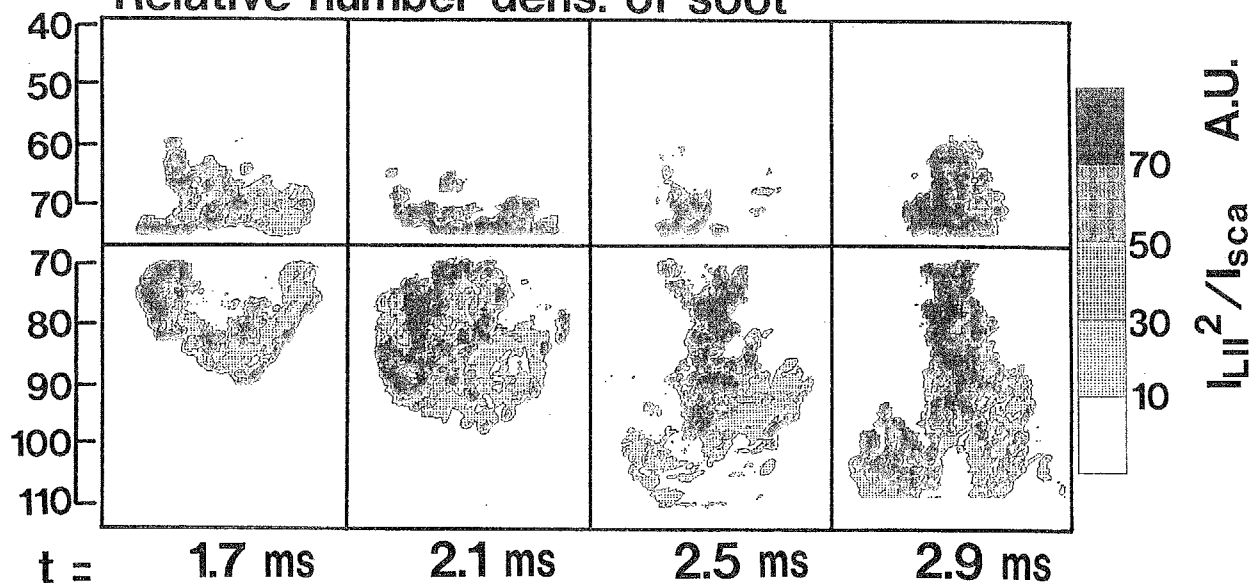
図 5 - 6 火炎断面内相対すす濃度分布 (上段)
