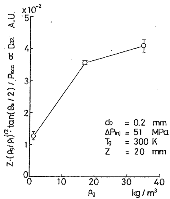
図 2 - 1 7 雰囲気気密度がパラメータ, \alpha , に及ぼす影響
