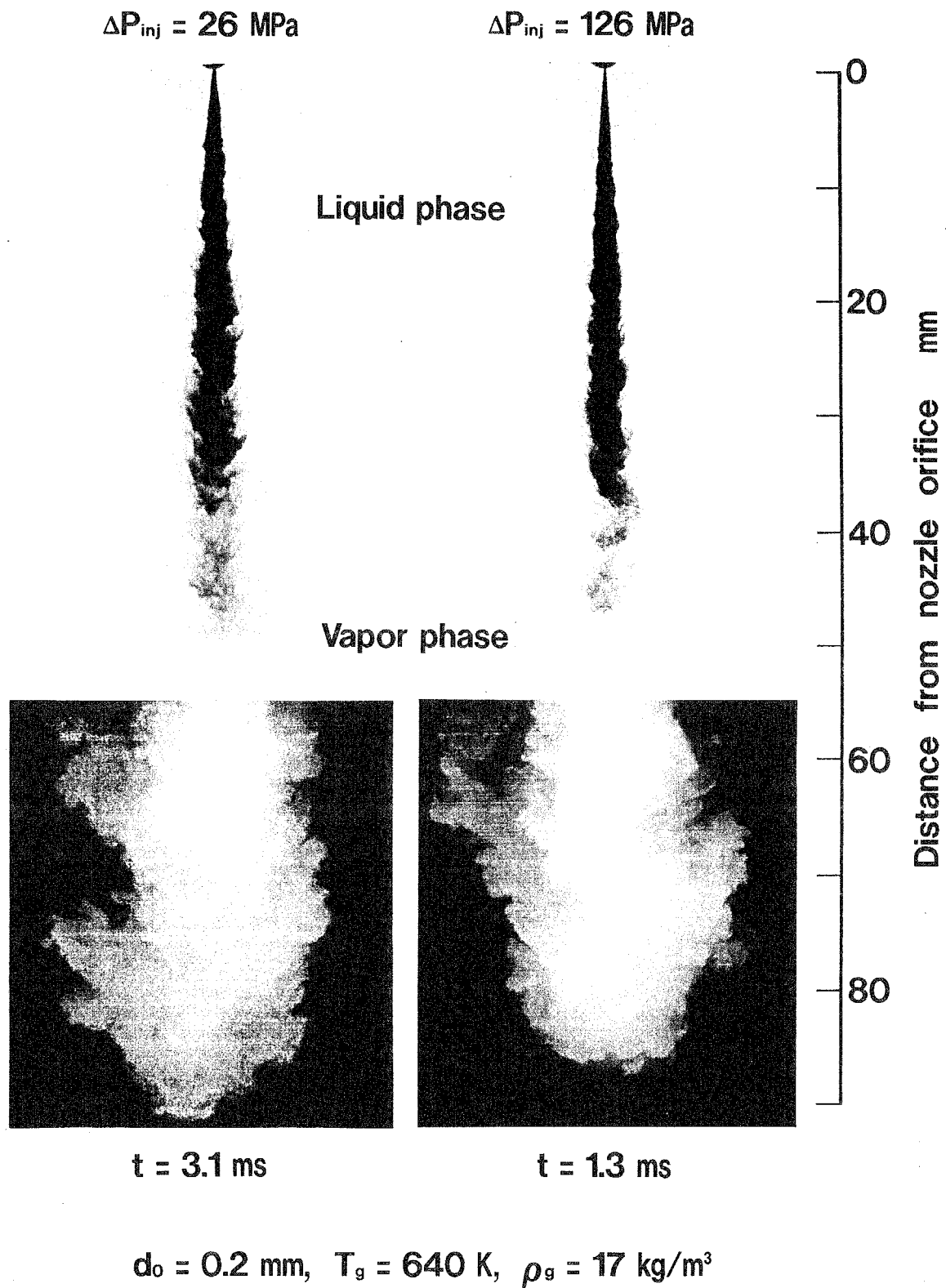
図 3 - 2 シリコンオイル粒子散乱光法により可視化された 蒸発噴霧断面内の燃料蒸気濃度分布（下）と 未蒸発液相部の背景散乱光写真（上）
