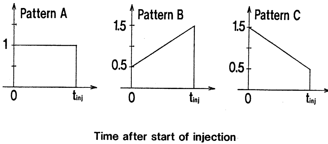
図 A-6 計算に用いた 3 種類の噴射率パターン
