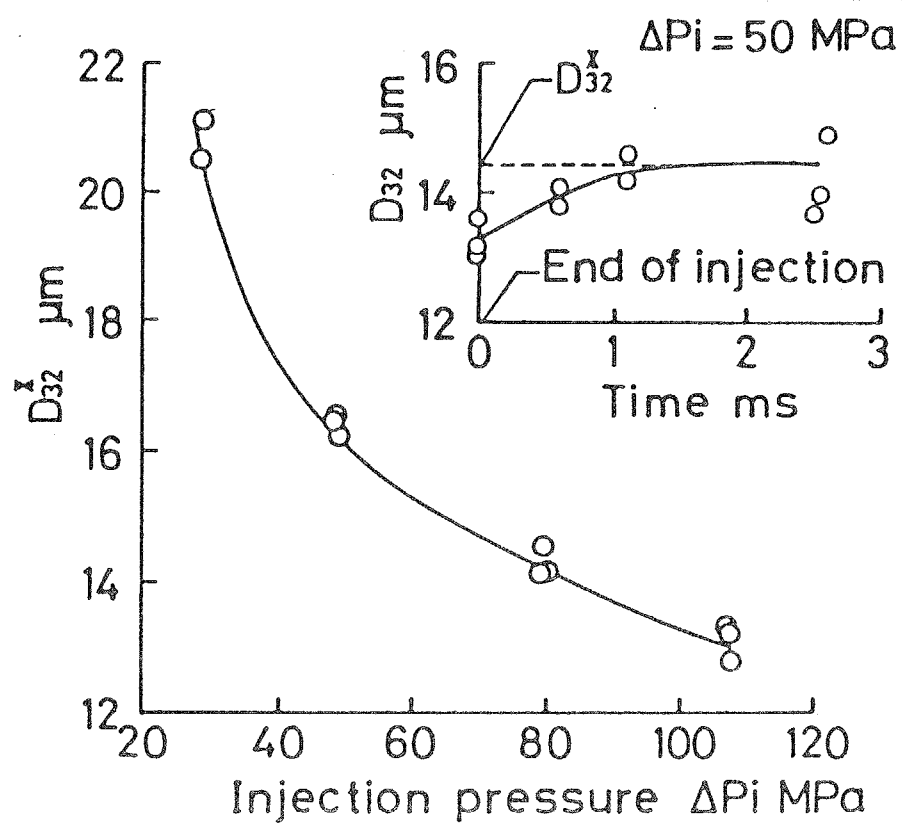
図 2-7 噴射圧力と噴霧全体に対するザウタ平均粒径
