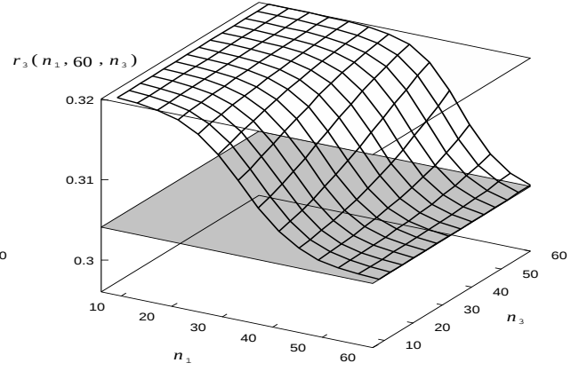
b: r_3(n_1, 60, n_3)
