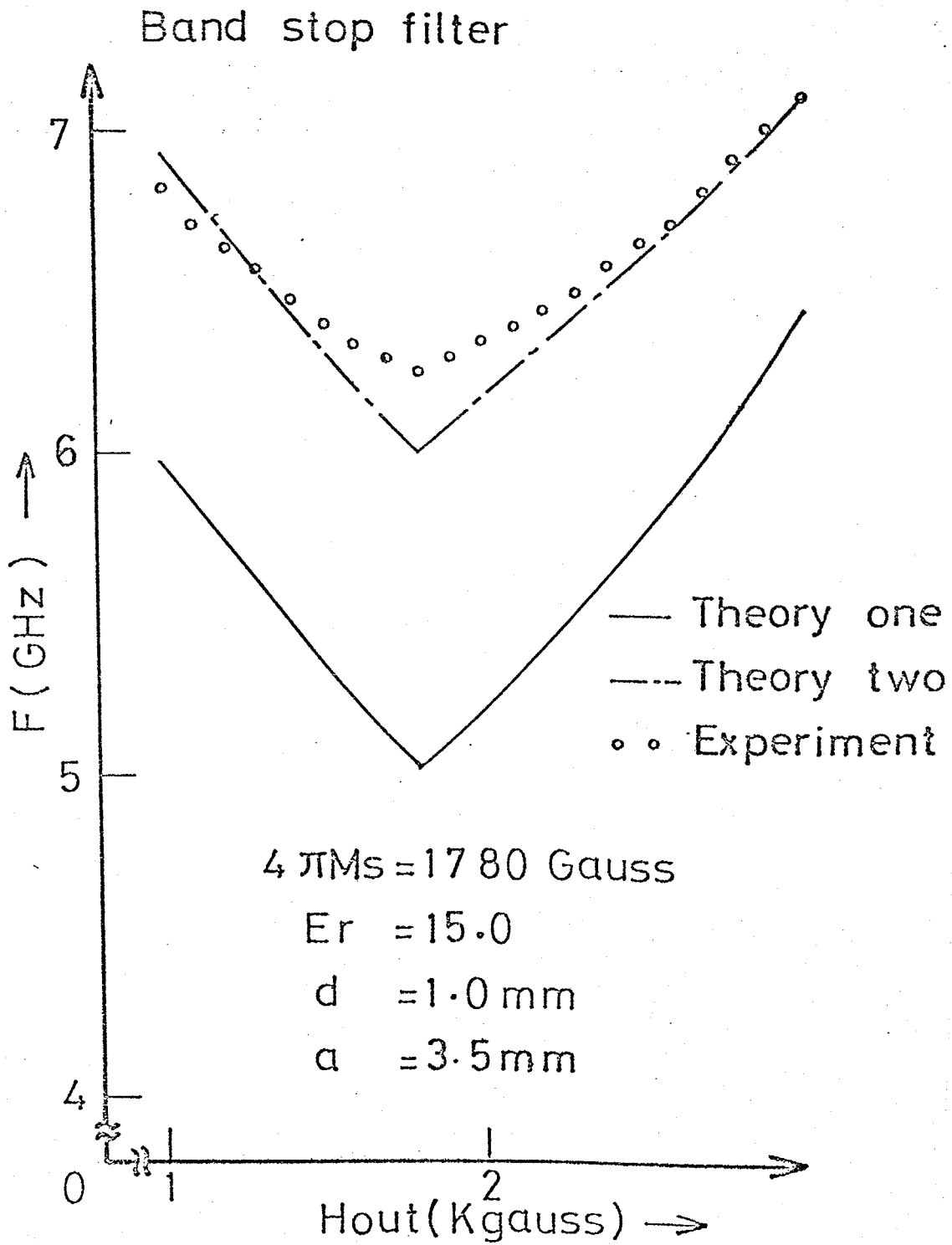
図 18. 同調特性
