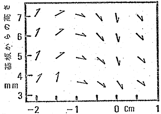
(a) 順方向
