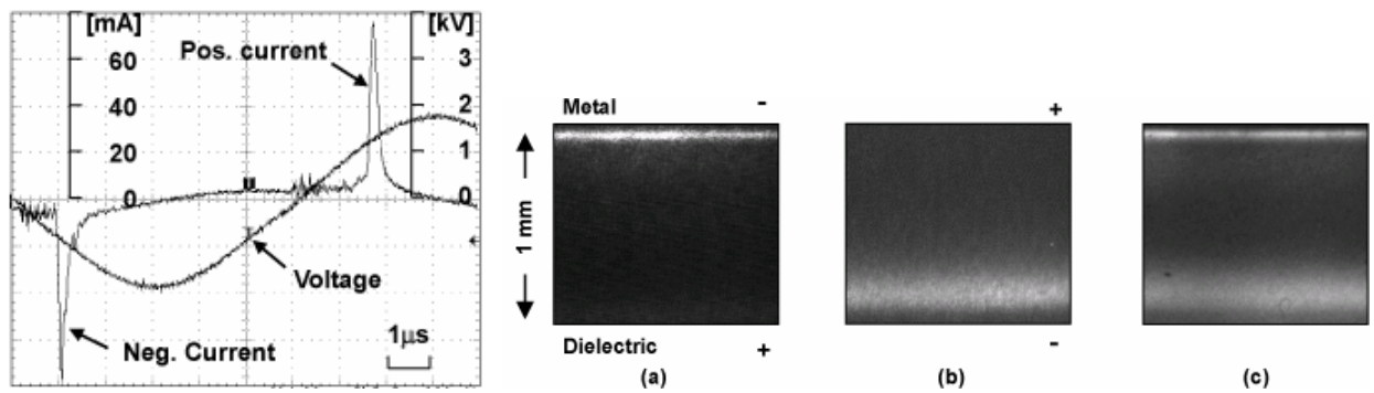
(a)負電流パルス (b)正電流パルス (c)正＋負パルス
