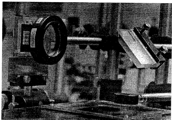
Fig. 3. 27 縮小光学系
