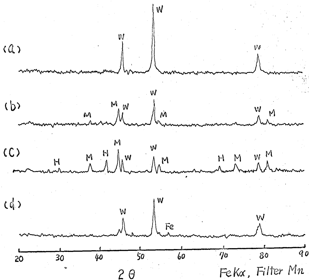
図18. 酸化鉄粉末X線回折図 1350°C, P_{\text{O}_2} = 10^{-9} atm
