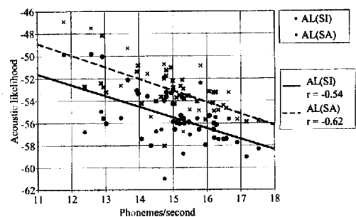
図 6 音響ゆう度と発話速度
