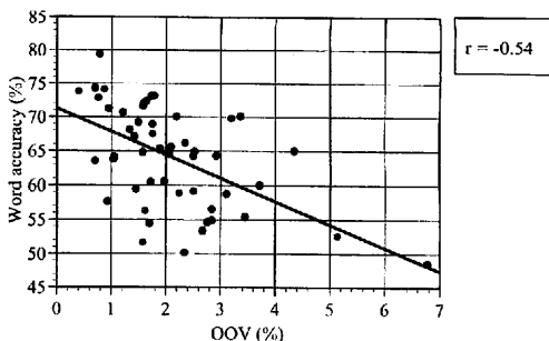
図 10 未知語率と単語正解精度
