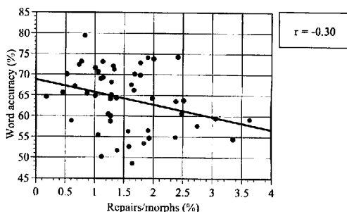
図 9 言い直し頻度と単語正解精度 (SI)
