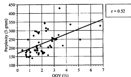
図 7 パープレキシティと未知語率
