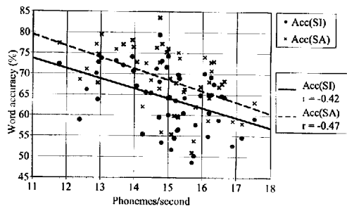
図 8 発話速度と単語正解精度
