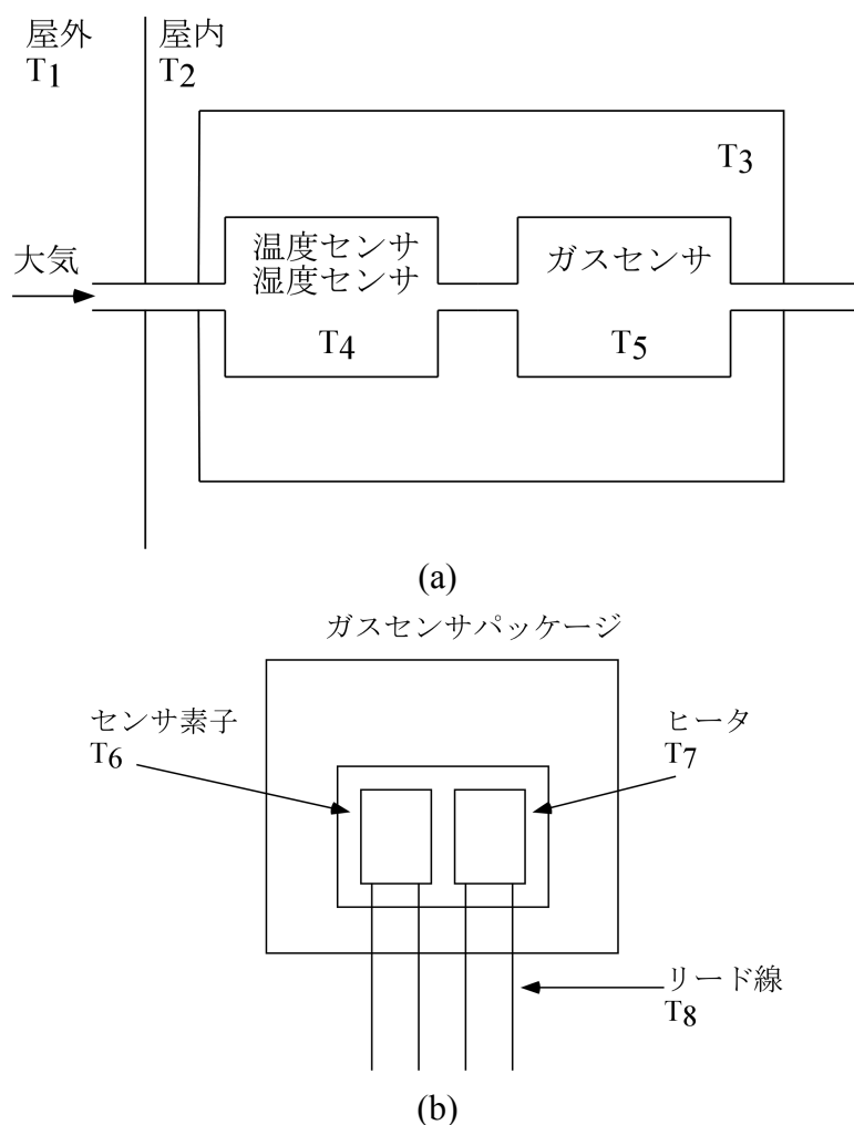
図 4.1 (a) NO 2 測定装置の概略、および(b) ガスセンサの構造
