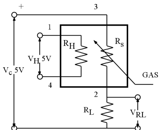
図 2.11 SP-61 測定回路
