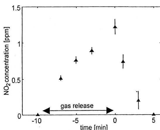
図 1.71 \text{NO}_2 測定結果
