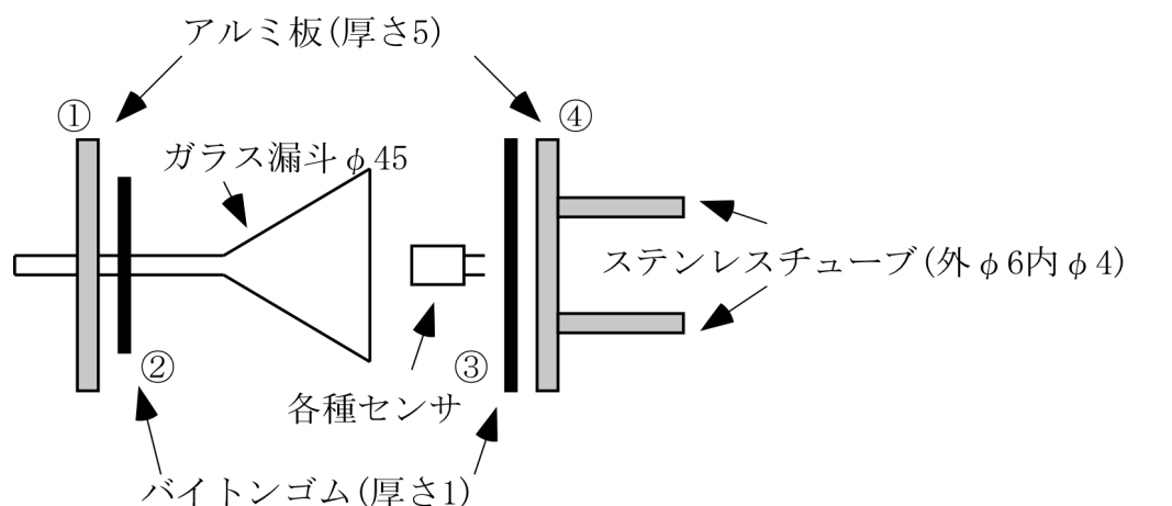
(a) センサセル上面図
