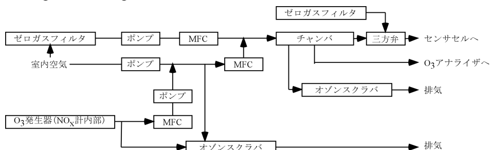
図 3.15 較正ガス発生装置
