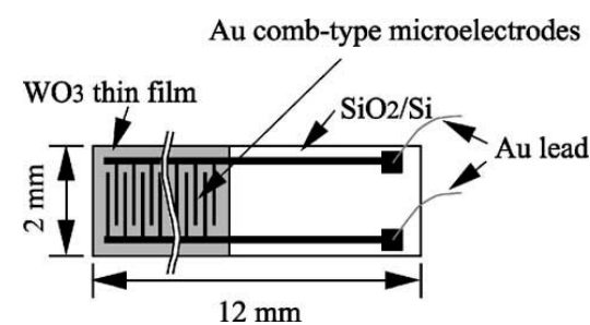
図 1.37 センサの構造
