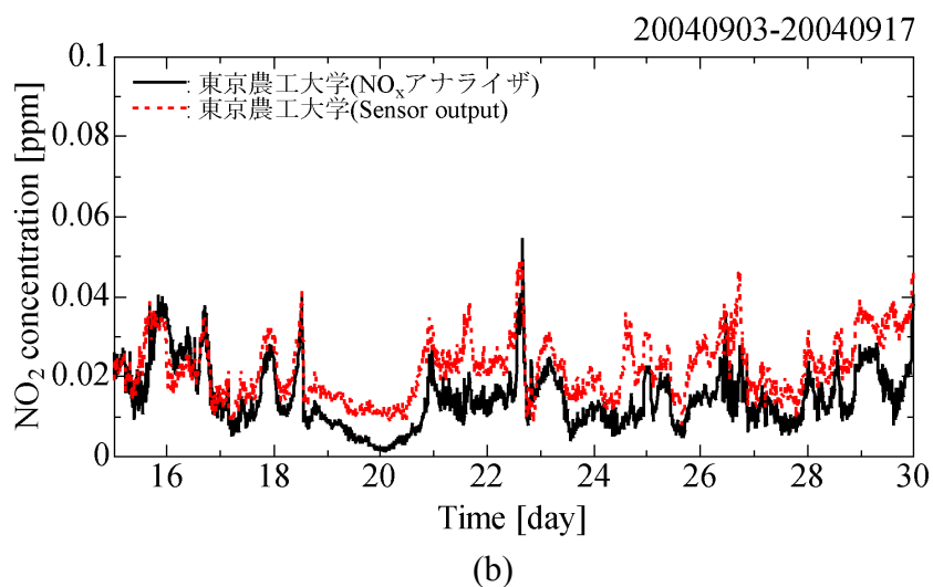
図 5.8 東京農工大学における大気中の NO_2 濃度測定結果
