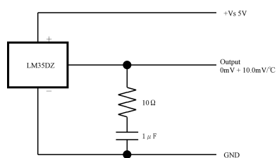
図 2.12 温度センサ測定回路
