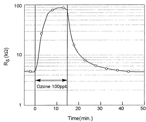
図 1.50 O_3 に対する応答スピード
