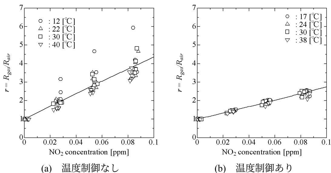
図 4.6 ガスセンサの \text{NO}_2 応答特性
