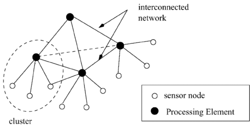
図 1.76 ネットワークの構造[90]
