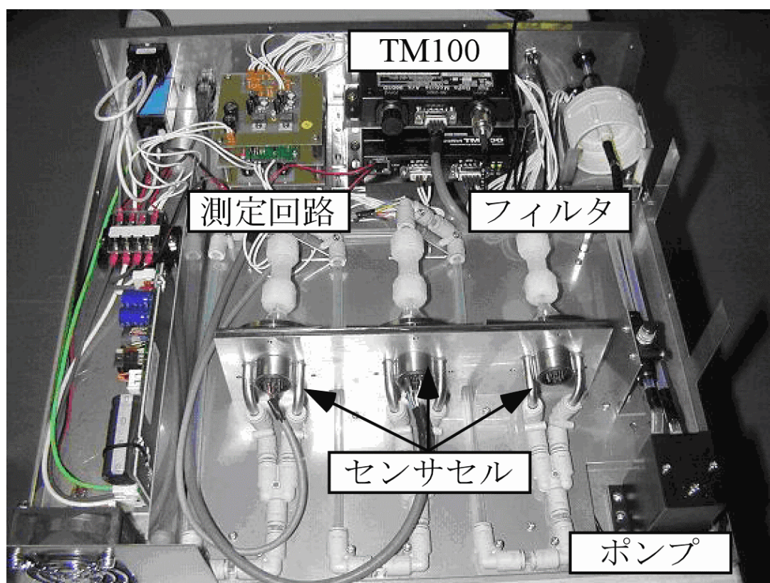
図 2.18 無線通信機能を搭載したガスセンサシステムの写真
