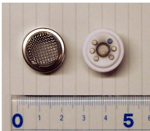
図 2.10 SP-61 の写真
