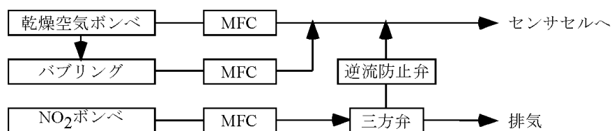
図 3.1 校正ガス発生装置
