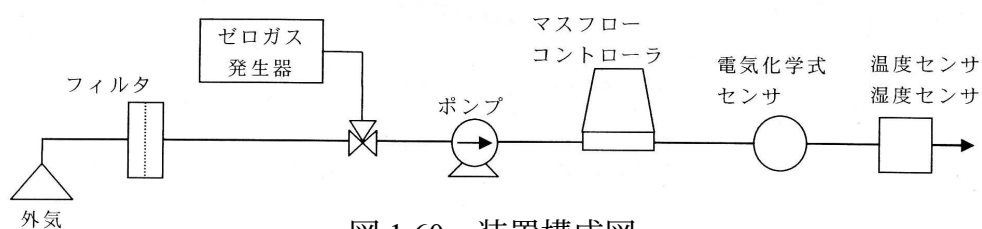
図 1.60 装置構成図
