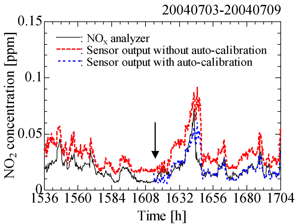
図 6.9 周辺測定局の測定値を用いた再校正の効果
