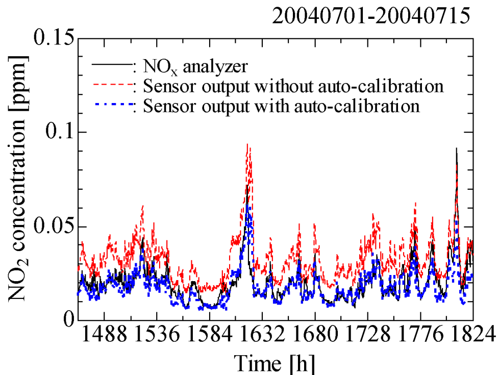
図 6.10 大気中の NO 2 濃度の測定結果
