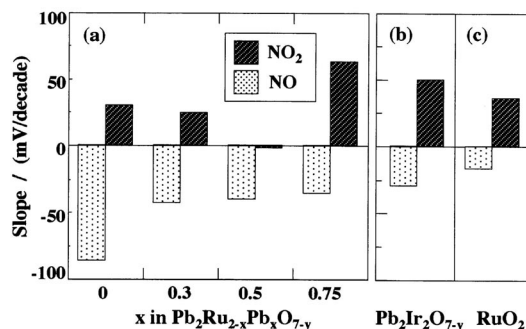
図 1.59 \text{NO}_x に対する応答
