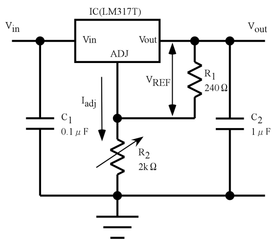
図 2.14 3 端子可変レギュレータ回路
