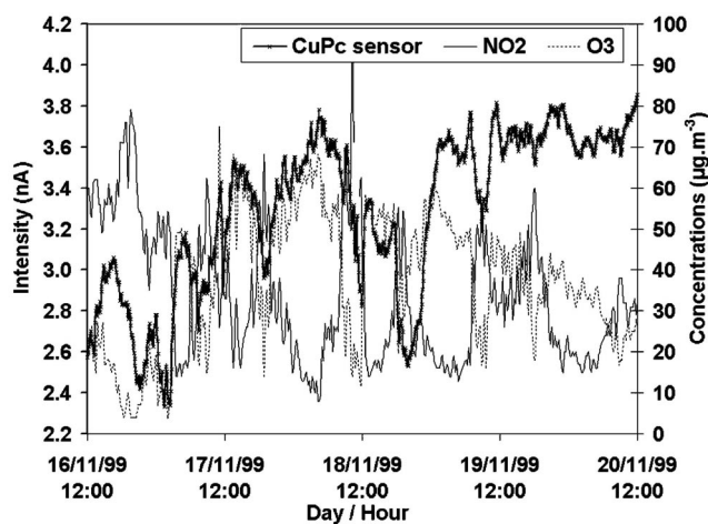
図 1.55 フィールド測定結果
