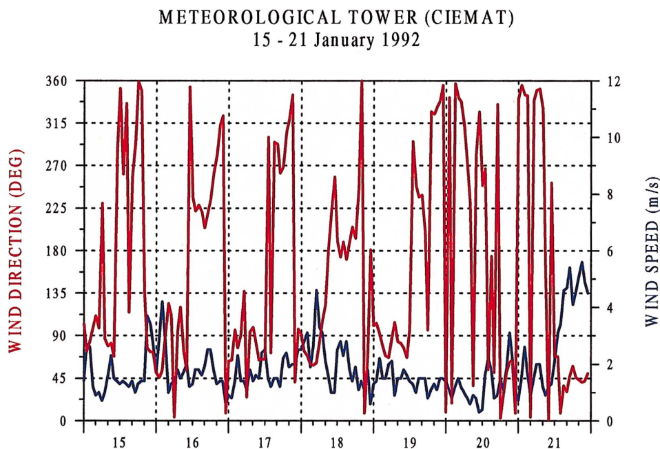
図 1.27 風向と風速の測定結果
