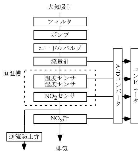
図 3.2 NO 2 センサ初期校正装置
