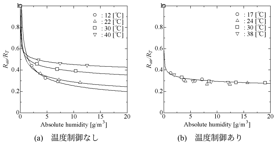
図 4.4 ガスセンサ抵抗の絶対湿度依存性
