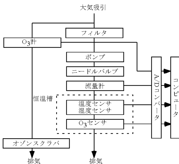
図 3.16 O 3 センサ較正装置
