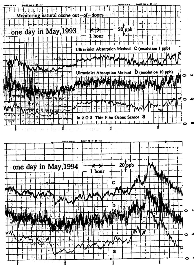
図 1.44 O_3 長期測定結果
