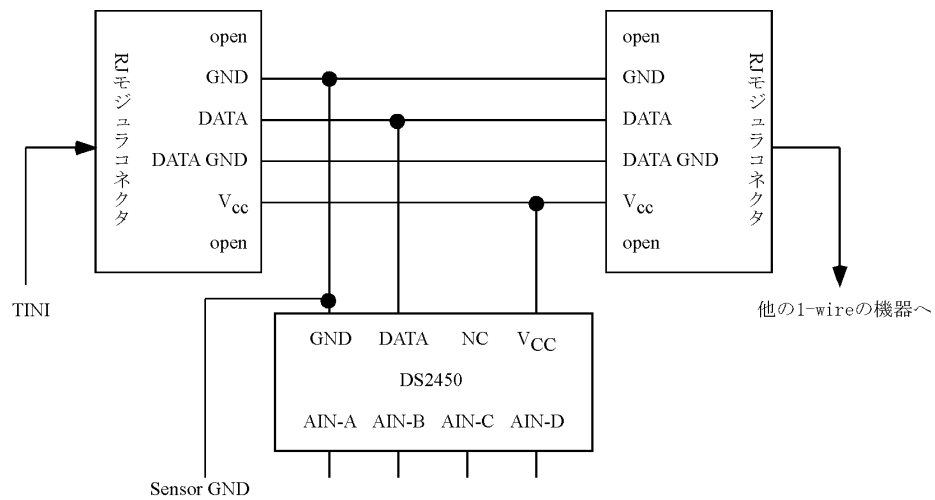
図 2.15 A/D コンバータの回路図
