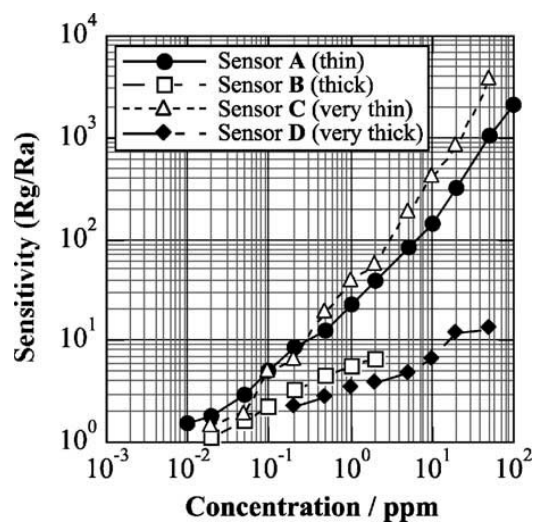
図 1.38 \text{NO}_2 に対する応答特性
