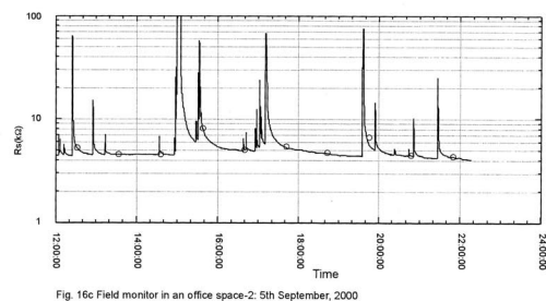
図 1.52 コピー室におけるモニタリング結果
