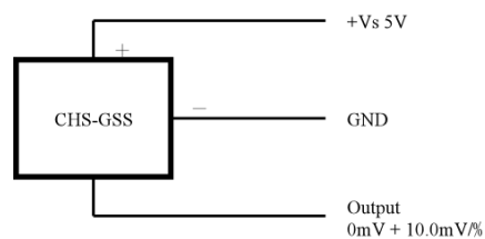
図 2.13 湿度センサ測定回路
