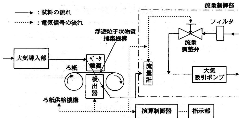
図 1.3 ベータ線吸収法の構成例[13]
