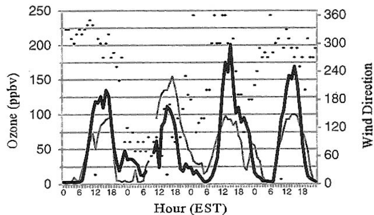
7/29 7/30 7/31 8/1 図 1.36 O 3 濃度と風向の時間推移
