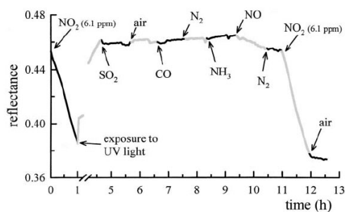
図 1.69 その他ガスに対する応答
