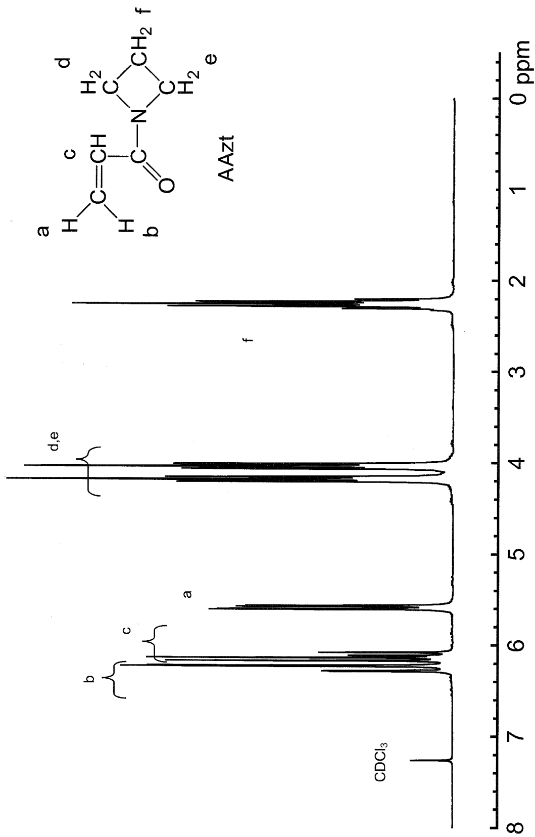
Figure 3-2-4. ^1\text{H} NMR Spectrum of AAzt.
