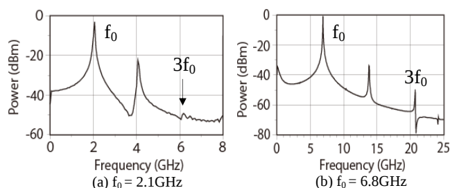
図 3 出力波形
