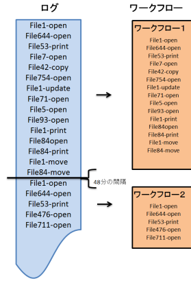
図 8 比較手法：ファイル及びタスクを抽象化せずに抽象ワークフローを抽出する例
