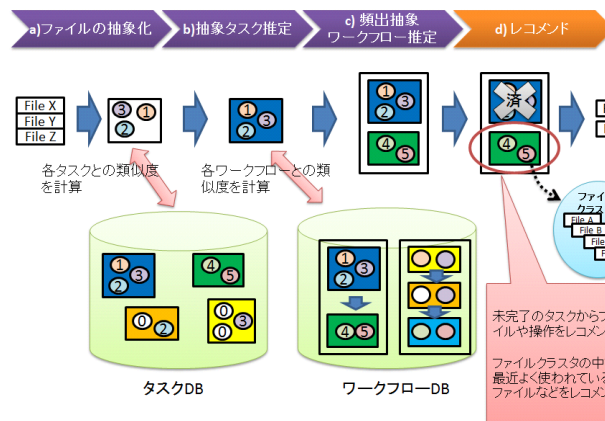
図 6 レコメンデーションを行う例
