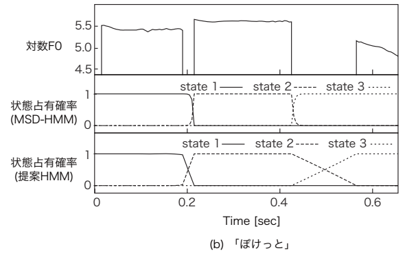
Fig. 1 中高型単語における状態占有確率の時間変化
