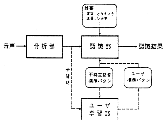
図 1 方式構成
