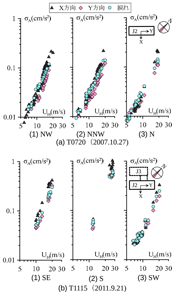
図2 風速による加速度の標準偏差の変化
