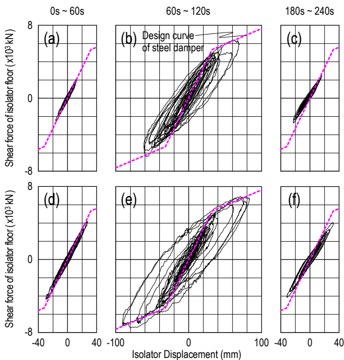
Figure 12. Hysteresis of isolator floor (a) ~ (c) : X-direction, (d) ~ (f) : Y-direction
