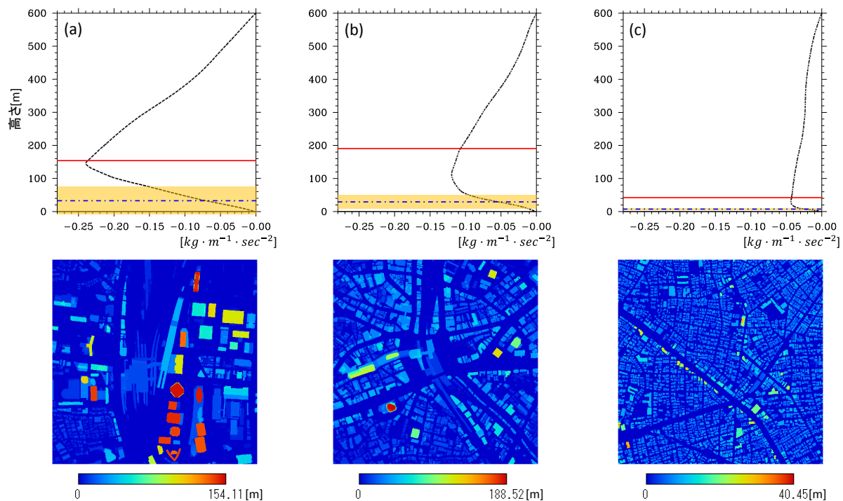
図-3 特徴的な運動量フラックスの鉛直プロファイル及び建物高さのコンター図
