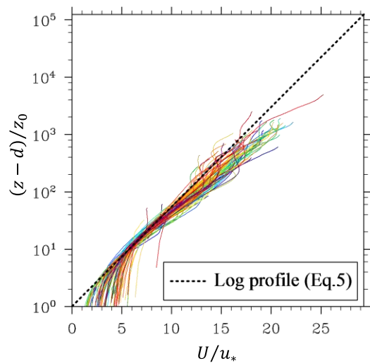
図-2 主流方向風速の対数分布
