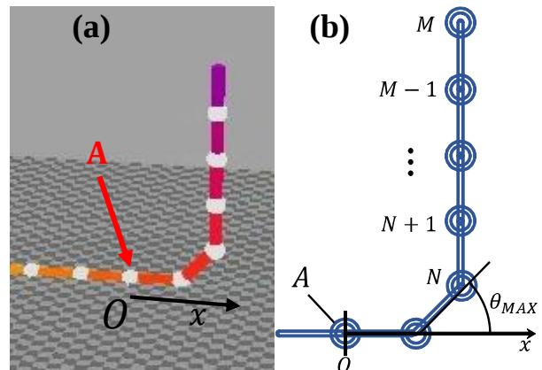
図2 垂直持上げの外観
