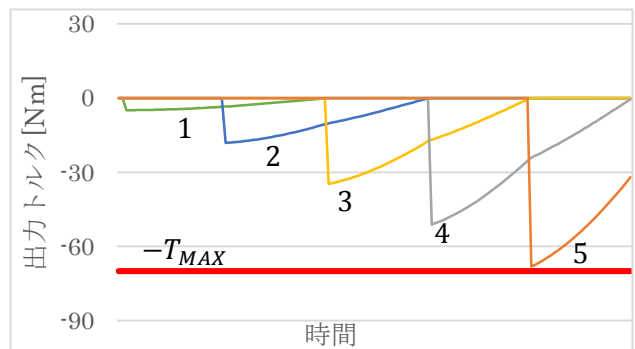
図 6 垂直持上げのトルクの変化
