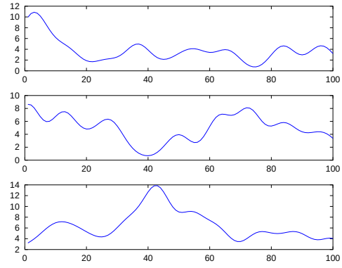
(d) Estimated signals \mathbf{A} (FastGRBF, SIR= 15.1 dB, \text{SIR}_M=10.7 dB)
