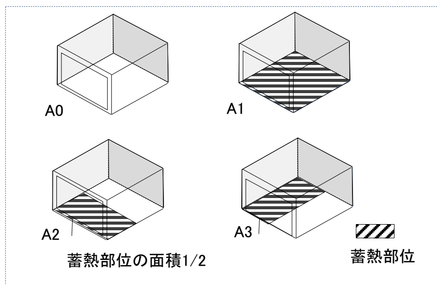
図 4-11 居間における蓄熱部位配置のパターン
