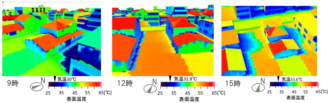
[B]平均放射温度分布(生活空間高さ1.5m)
