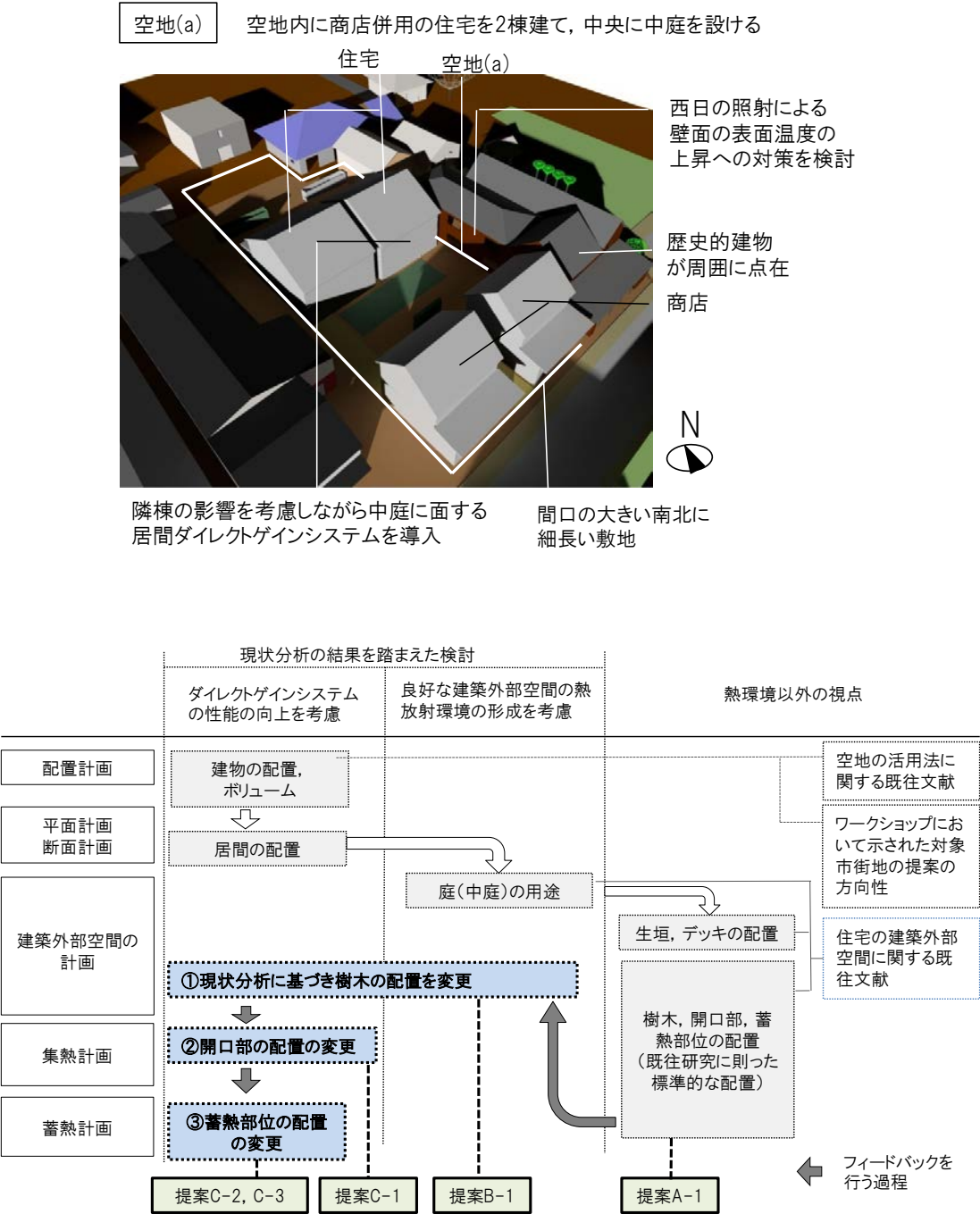
図 5-2 空地 (a) における提案の概要と提案の流れ
