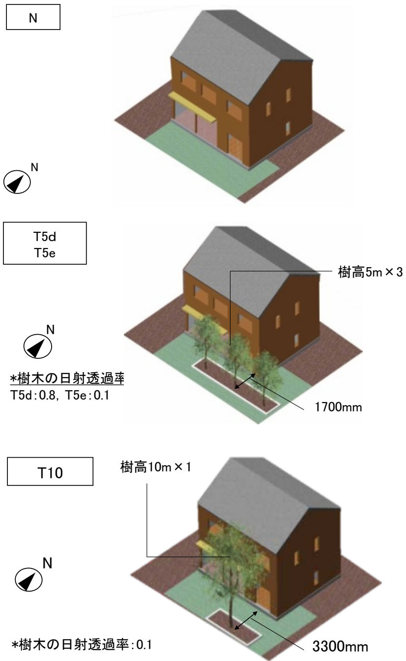
図 4-10 建築外部空間のパターン
