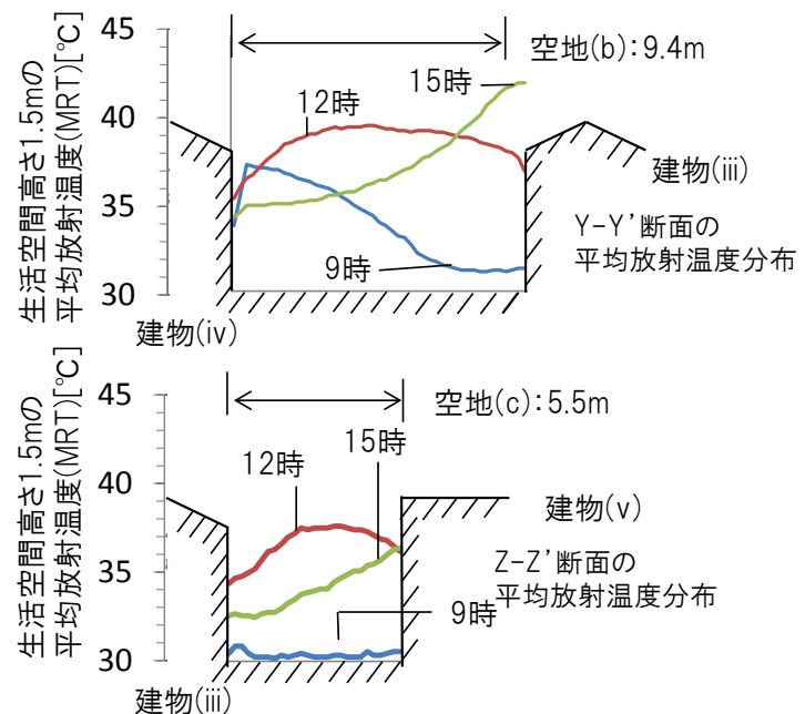
図 2-12 東西の間口の異なる空地 (b), (c) の表面温度分布と生活空間高さ 1.5m の平均放射温度
