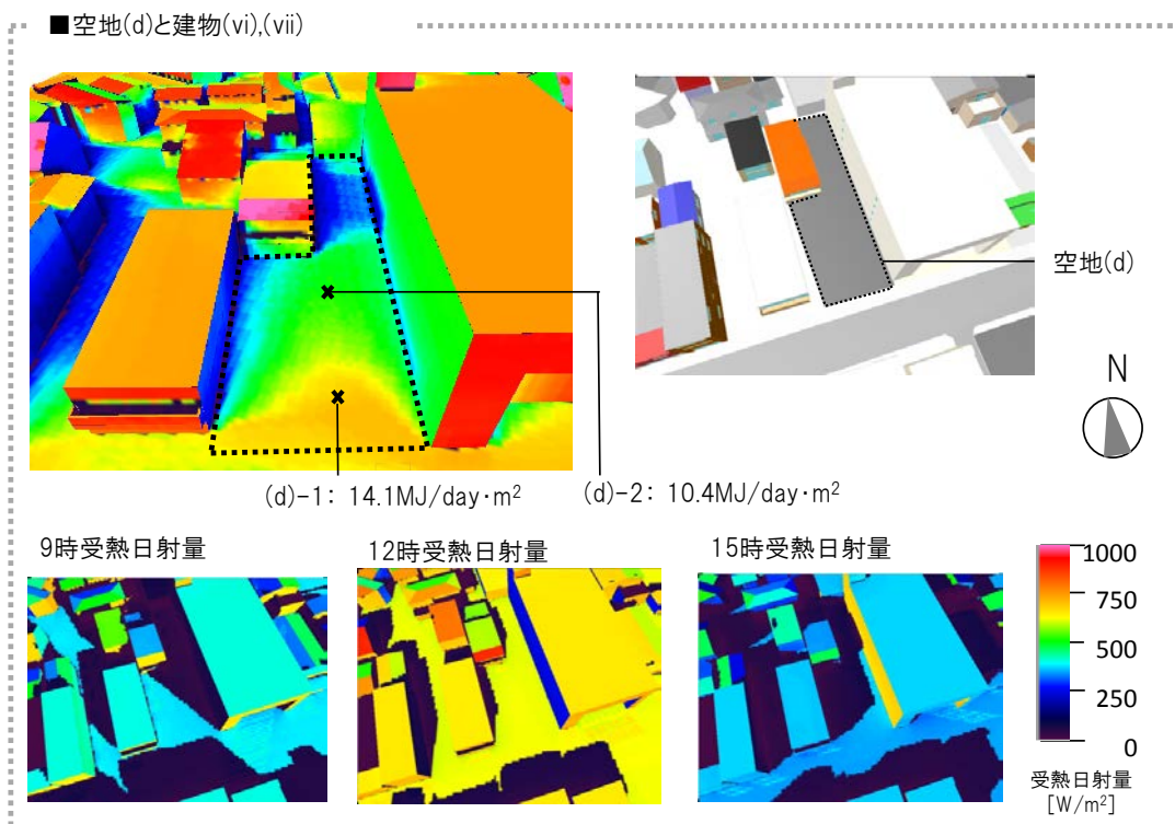
図 2-8 空地 (b), (c), (d) 内における冬季の受熱日射量分布
