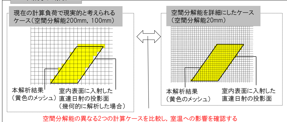
図 4-2 提案した性能予測方法に存在する誤差要因とその室温への影響の解析方法
