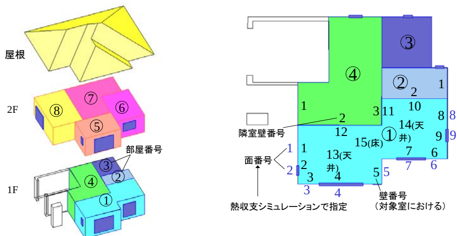
図 3-5 本研究における各シミュレーションの空間モデル
