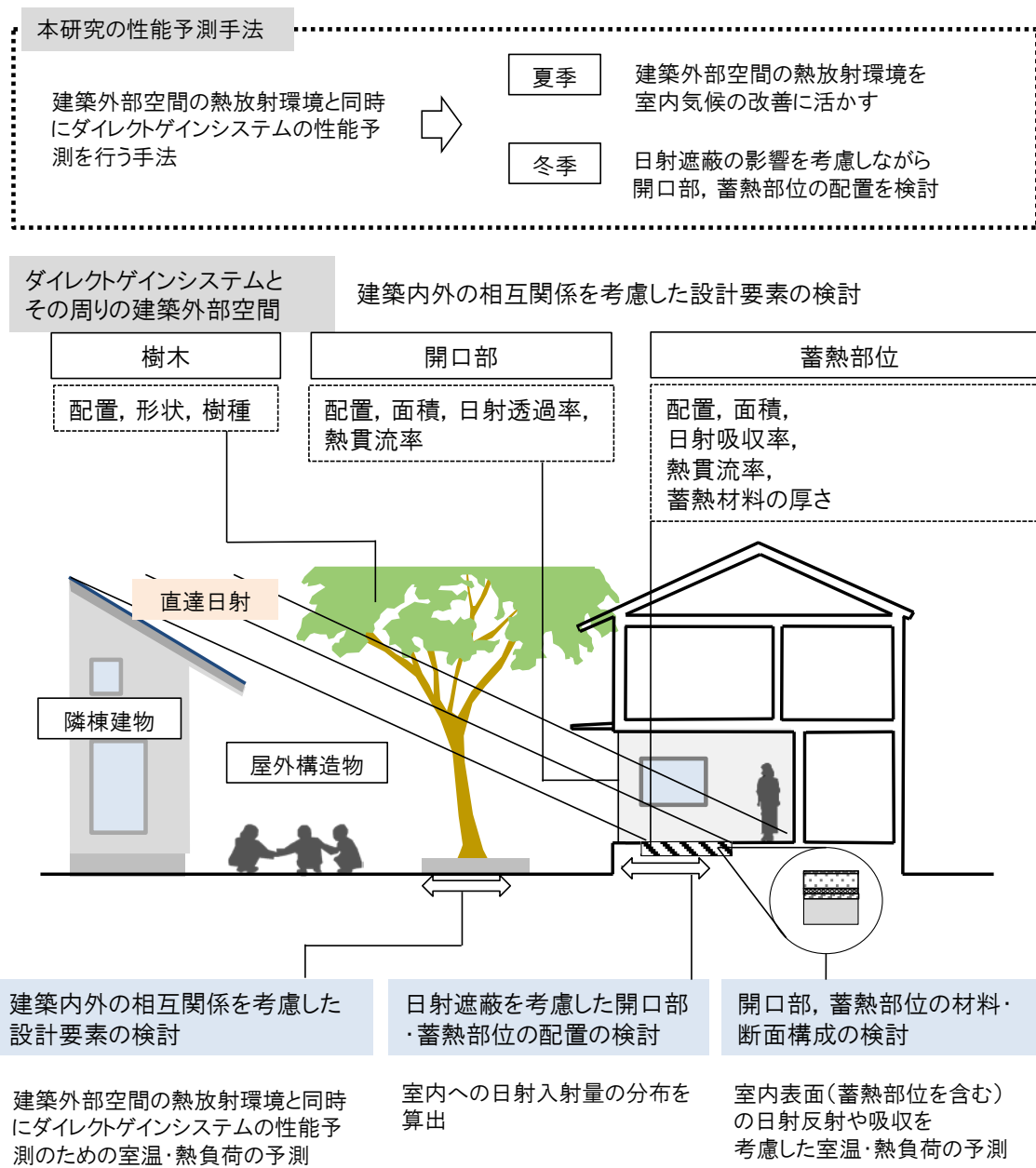
図 3-1 ダイレクトゲインシステムの性能予測のための要件
