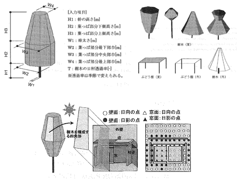
図 3-3 樋口らのモデルにおける日射遮蔽の取り扱い
