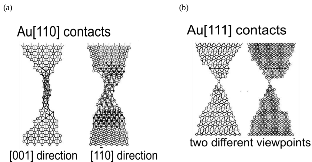
Fig.2. 6 : 分子動力学計算によって得られた，変形過程のスナップショット．(a)Au[110]接合，(b)Au[111]接合 M. Sørensen, M. Brandbyge, and K. Jacobsen (1998) [6].
