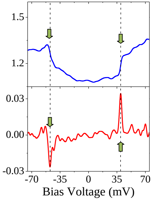
Fig.6.4 : 水素吸着時における Co 単原子接合の振動スペクトル.
