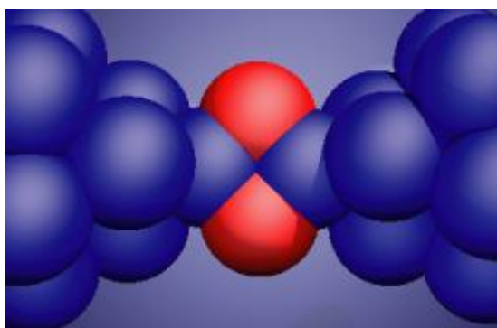
Fig. 6 : 水素を吸着した Co 単原子接合のモデル図. 青玉 : Co もしくは Pt 原子, 赤玉 : H 原子.
