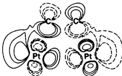
Fig.7.11 : \text{Pt}_2\text{C}_2\text{H}_4 クラスターの LUMO の一定電子密度の等高線図 J. A. Horsley, J. Stöhr, and R. J. Koestner (1985) [9].
