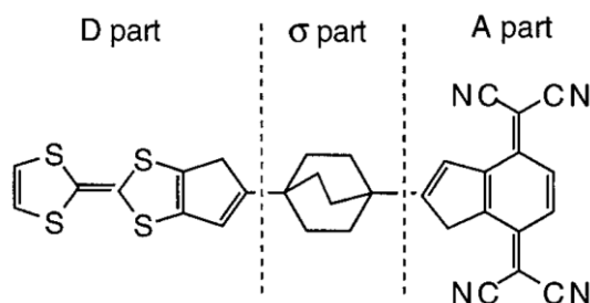
Fig.1.2 : D-σ-A 分子 A.Aviram and M. A. Ratner (1974) [2].
