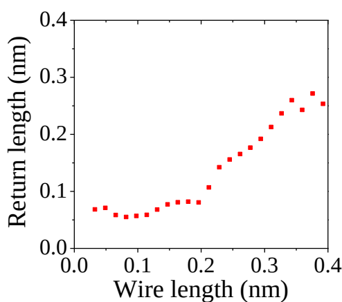
Fig.6. 3: Co 単原子接合の伸張距離の評価. (a)レンジスヒストグラム(b)伸張距離に対する平均戻り長.
