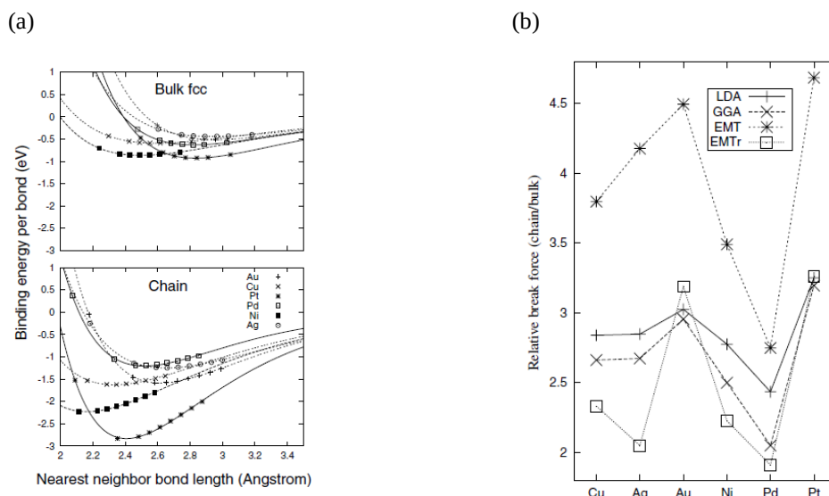
Fig.6. 1. : (a) 原子間の結合エネルギーと(b) バルクにおける結合の破断に必要な力とワイヤの場合の力の比の計算結果 S. Bahn and K. Jacobsen (2001) [10].
