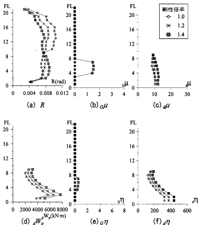
図10 剛性の増大による応答変化 ( \alpha_y=0.06 , 耐力 1.2 倍)
