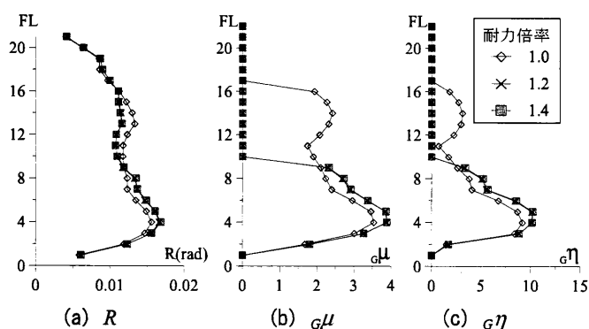
図4 耐力の増大による応答変化(剛性1.0倍)
