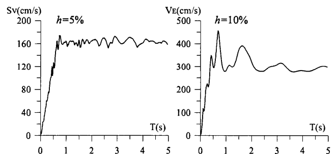
(a)速度応答スペクトル (b)エネルギースペクトル
