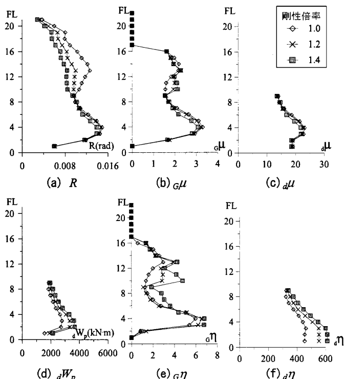
図9 剛性の増大による応答変化 ( \alpha_y=0.02 , 耐力 1.0 倍)
