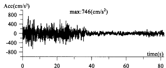
図2 加速度時刻歴波形
