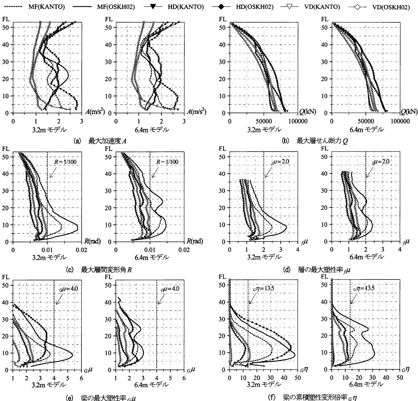
図5 応答性状の高さ方向分布
