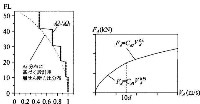
図1 ダンパーのせん断力比分布 図2 粘性抵抗力
