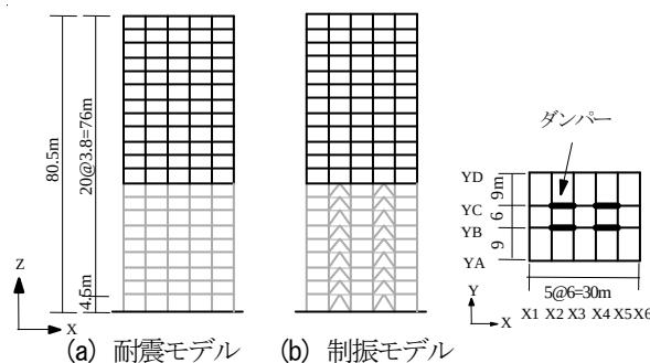
図 1 建物概要
