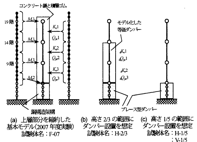
図1 実験条件と試験体名
