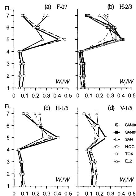
図2 各層が吸収したエネルギーの分担率
