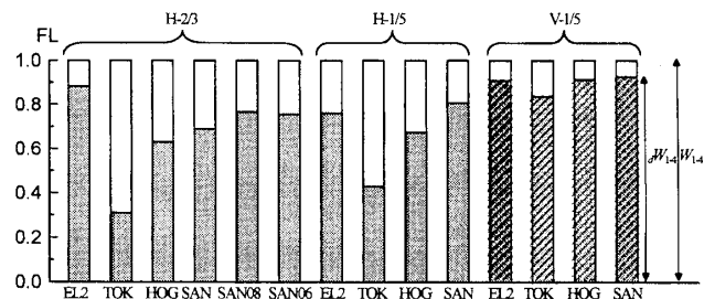
図3 ダンパーのエネルギー分担率
