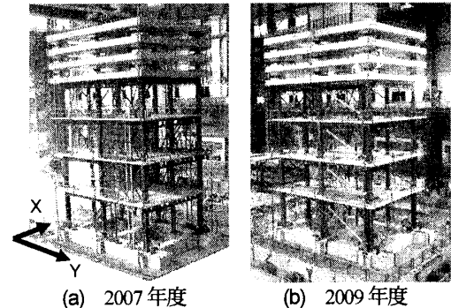
写真1 試験体写真
