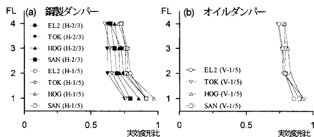
図4 ダンパーの実効変形比
