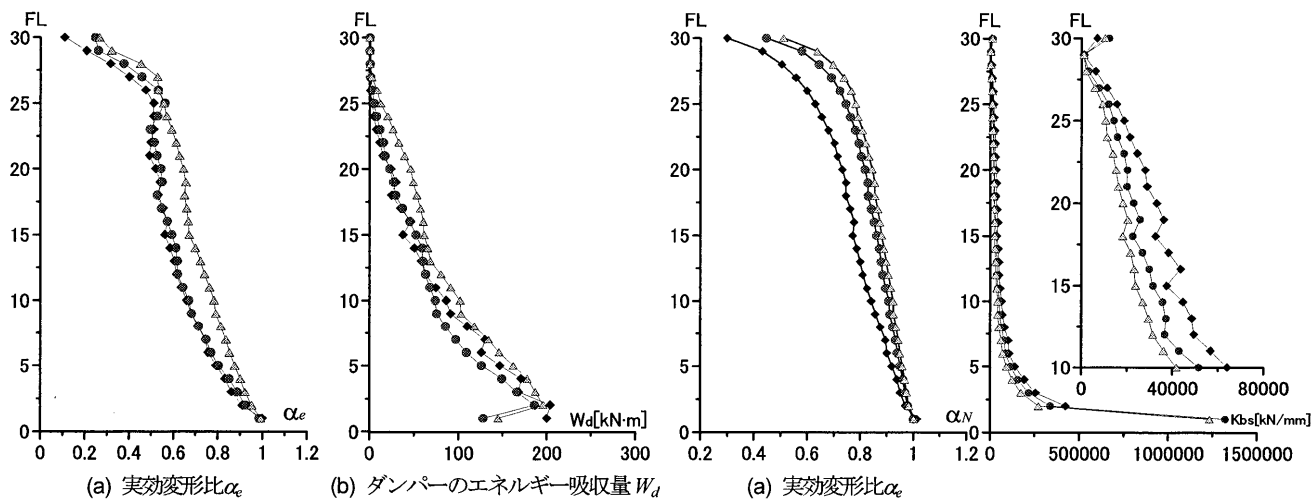
図2 架構別の高さ方向の応答分布および架構特性分布 (配置B)
