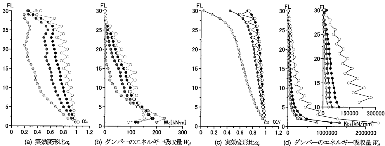
図3 配置別の高さ方向の応答分布および架構特性分布 (37H)
