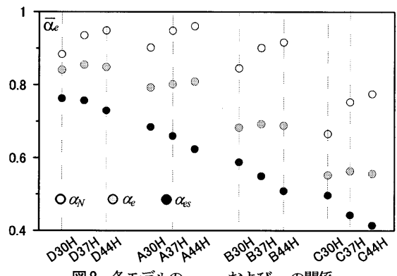
図8 各モデルの \alpha_N , \alpha_e および \alpha_{es} の関係
