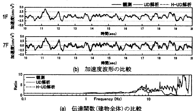
図9 上下応答解析結果(岩手県内陸南部)
