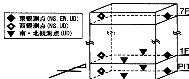
図1 観測点の配置図
