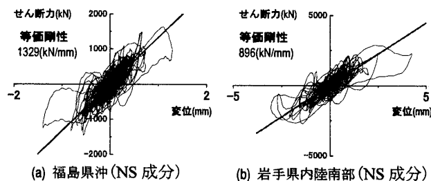
図3 免震層履歴曲線の比較
