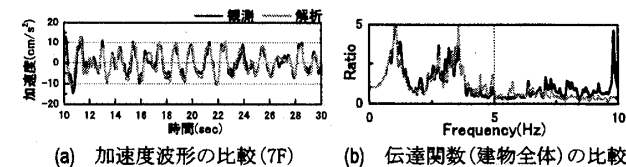
図8 水平応答解析結果(岩手県内陸南部NS方向)
