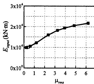
図 7 \mu_{rms} による E_{input} の変化
