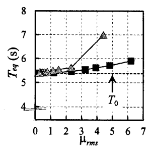
図 6 弾性周期と等価周期比較
