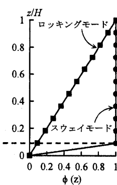
図 10 振動モード形概要
