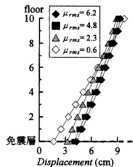
図 9 応答変位の標準偏差
