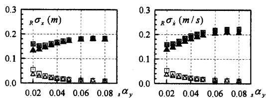
図 6 応答の予測値と時刻歴応答解析結果の比較
