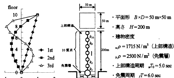
図1 上部構造モード分布 図2 弾塑性解析モデル概要
