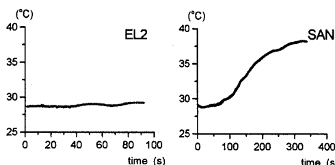
図9 オイルダンパー表面温度時刻歴
