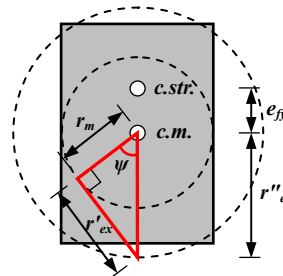
図4 モード比例荷重下と質量比例荷重下での等価弾力半径の比較
