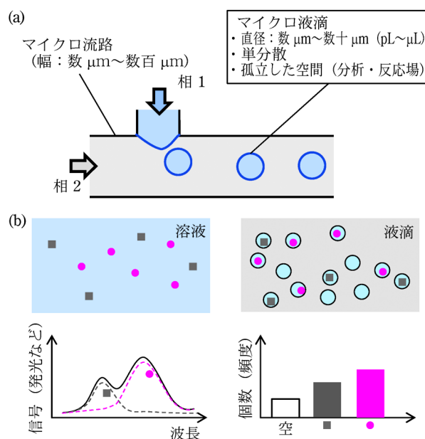
図1 (a) マイクロ流路中のマイクロ液滴の概観, (b) 溶液中の定量操作(左)と液滴を用いる定量(右)の比較
