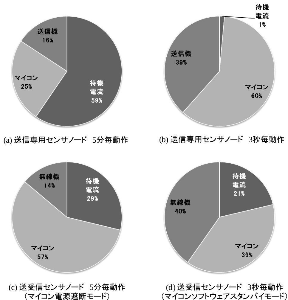
図 3-20 センサノードの平均消費電流における各ブロック電流の割合
