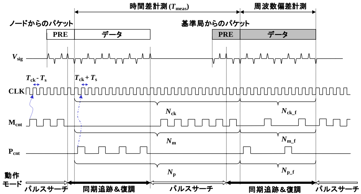
図 4-4 UWB-IR 受信機のタイミングチャート
