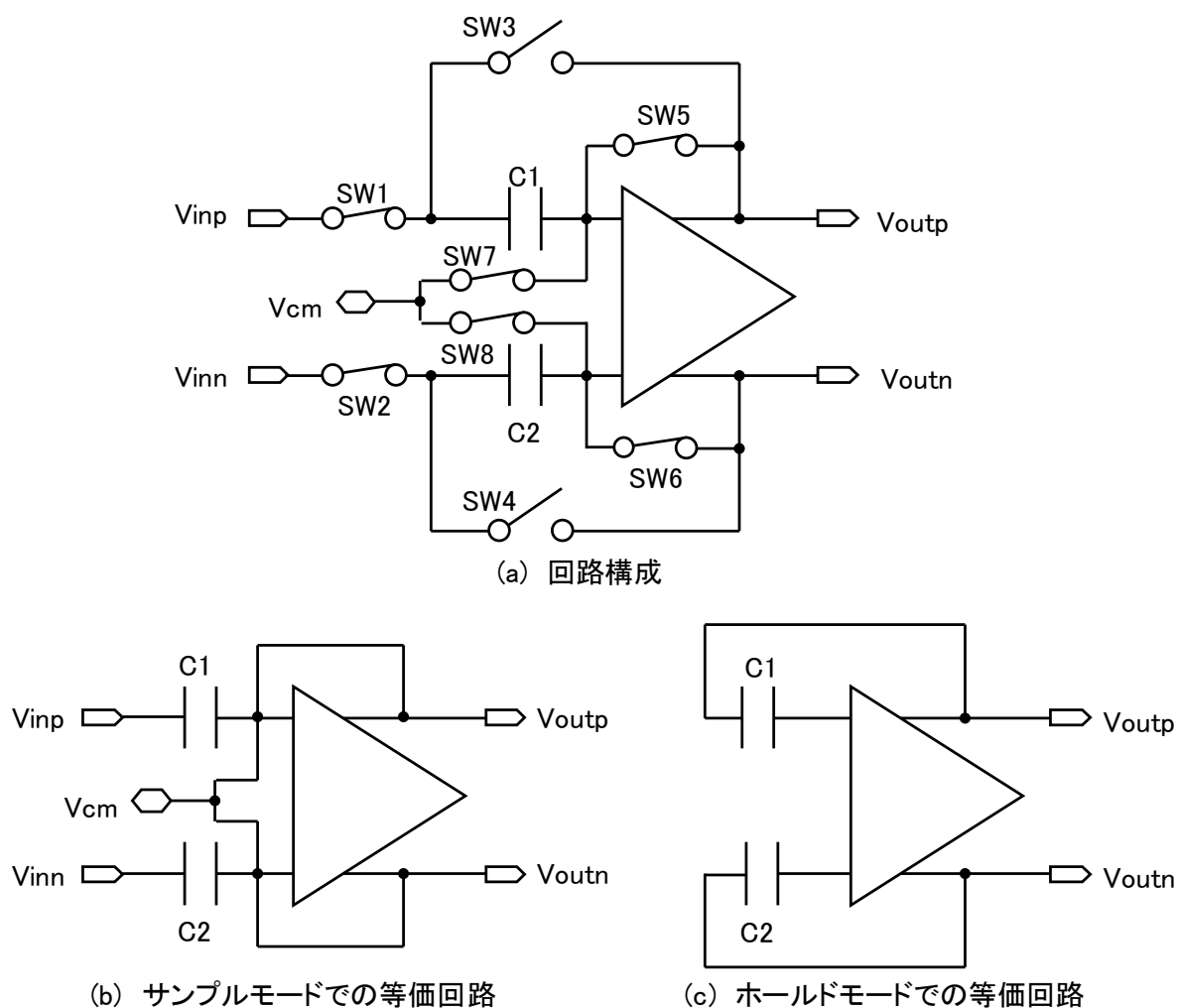
図 2-14 従来の S&H 回路に定電圧サンプリングを追加した回路
