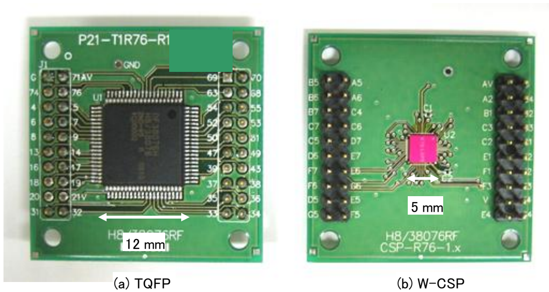
図 3-4 実装方式の比較
