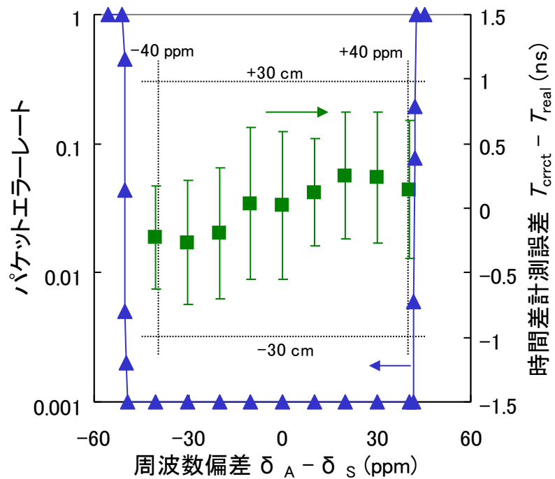
図 4-11 周波数偏差とパケットエラーレートおよび時間差計測誤差の関係
