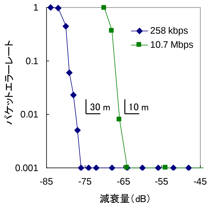
図 3-14 通信性能評価結果
