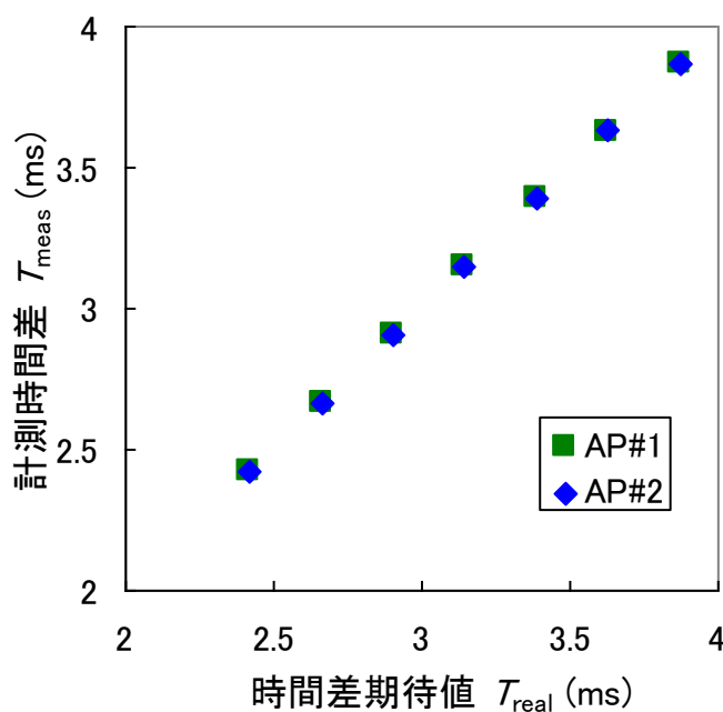
図 4-6 計測時間差と期待値との関係
