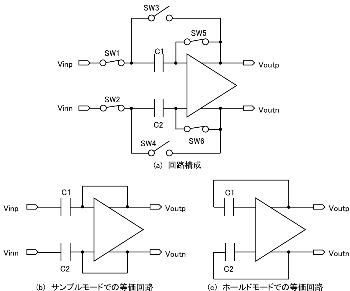
図 2-13 従来の S&H 回路
