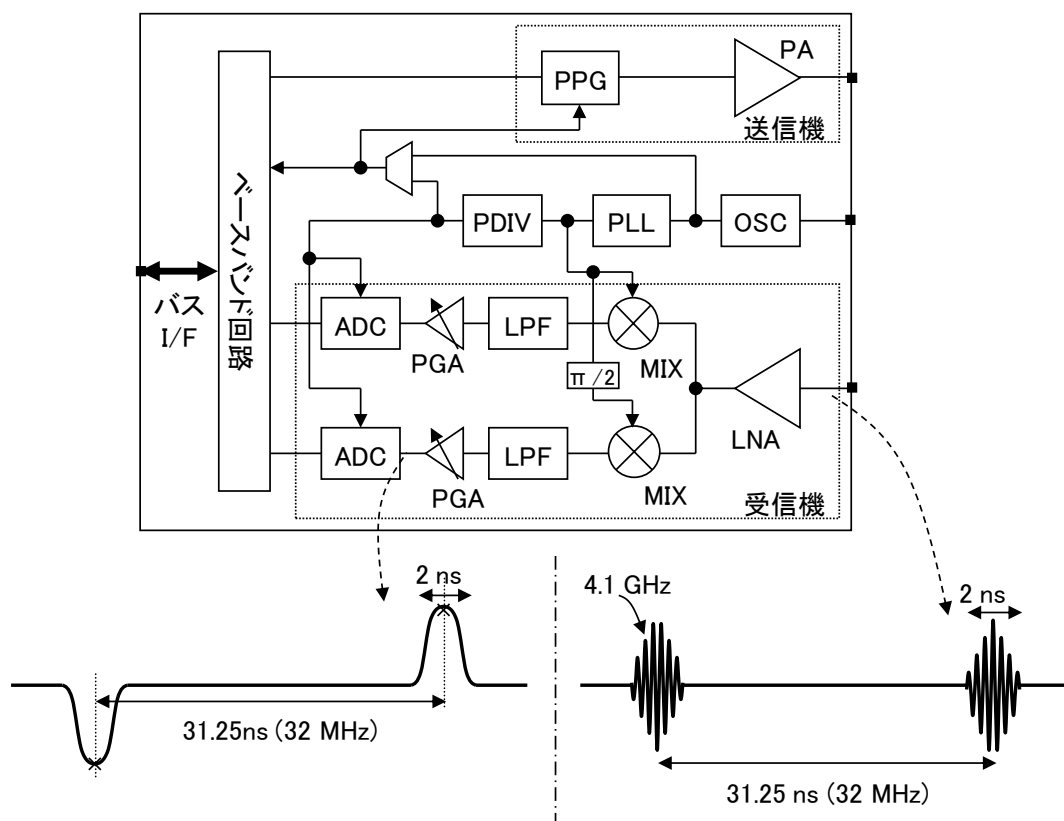
図 2-2 UWB-IR 通信 LSI のブロック図
