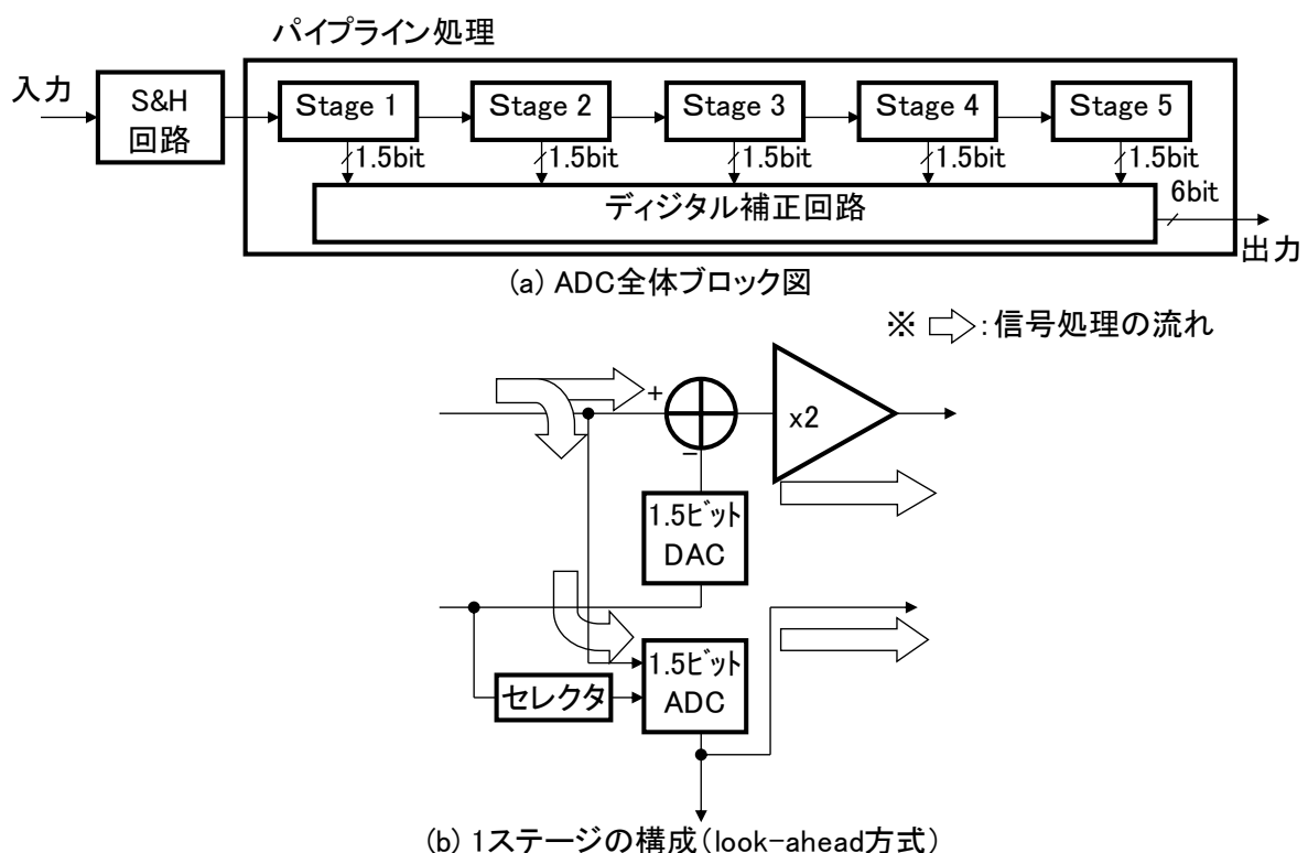
図 2-11 提案 ADC のブロック図
