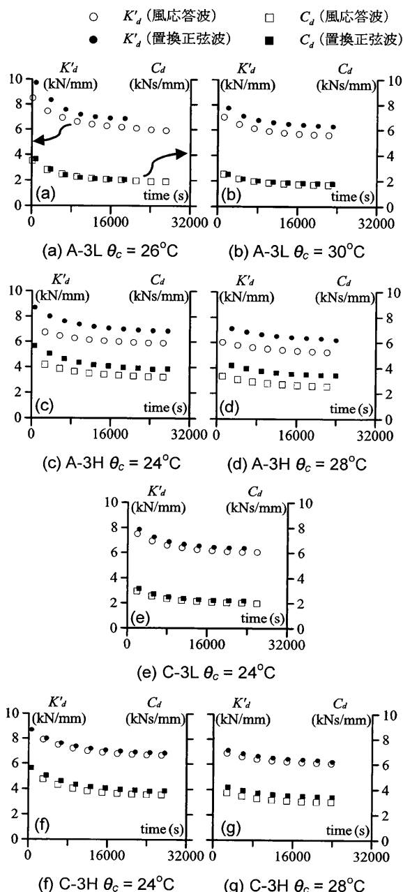
図 5 風応答波と置換正弦波での K'_d , C_d の変化
