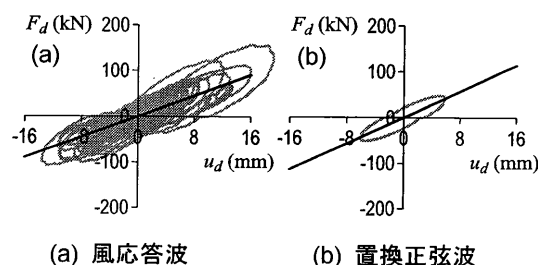
図 6 特定の 400 秒間における荷重-変形関係 (A-3H 室温 28°C)
