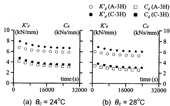
図2 A-3H, C-3Hにおける K'_d, C_d の変化
