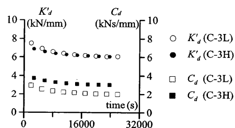
図3 \theta_c = 28^\circ\text{C} における K'_d, C_d の変化
