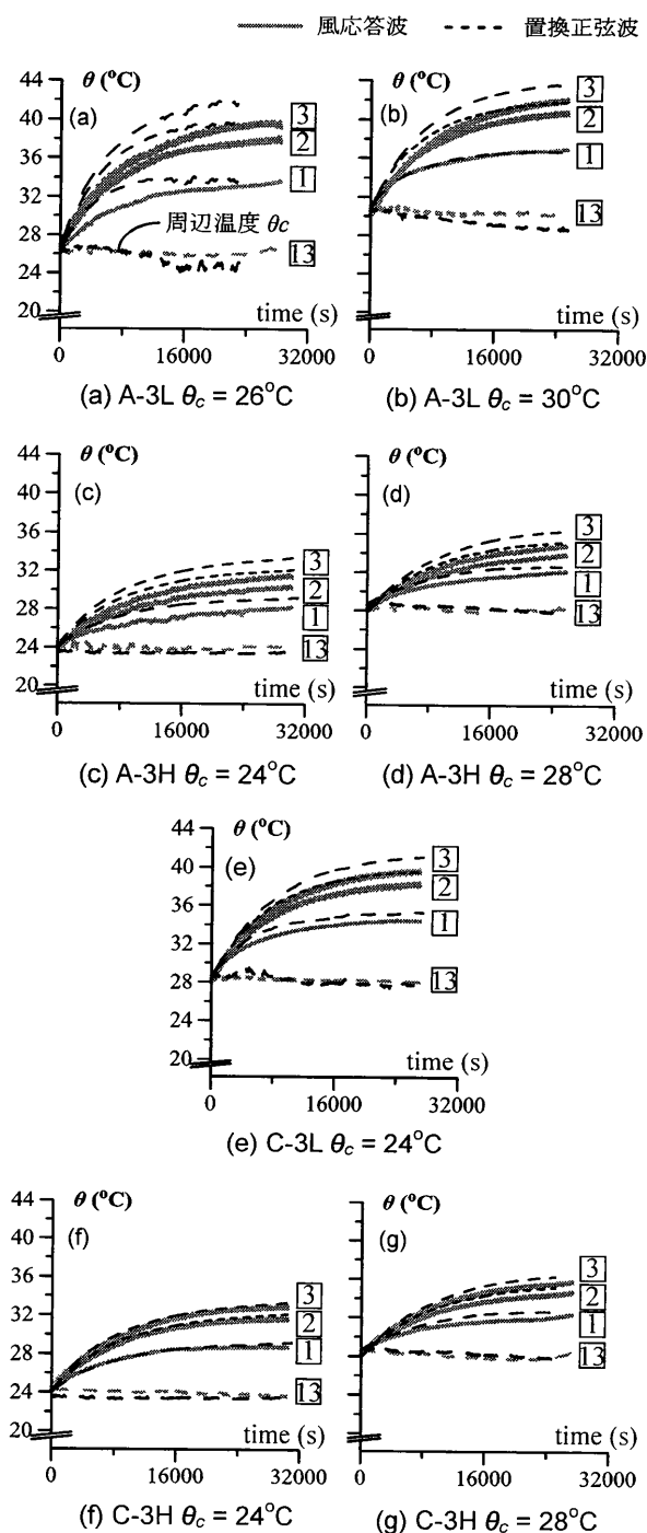
図 4 B-B'断面左側上段 風応答波と置換正弦波の温度時刻歴
