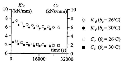
図1 A-3L 長時間風応答波実験での K'_d , C_d の変化
