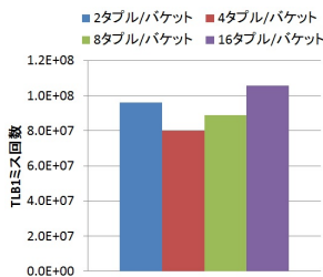
図 19 TLB1 ミス
