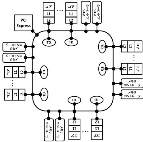
図 7 Xeon Phi のアーキテクチャ簡略図
