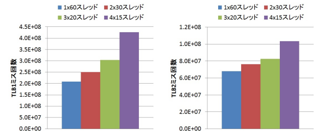
図 15 TLB1 ミス
