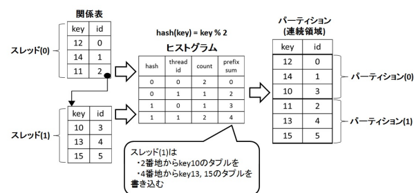
図 5 radix-partitioning の例
