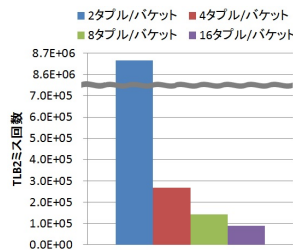
図 20 TLB2 ミス
