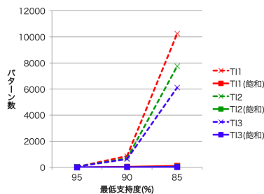
図 5 抽出数 (右白内障)
