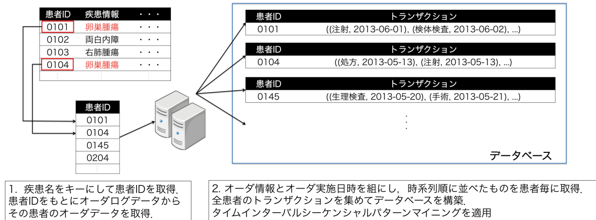
図 1 本手法の概要
