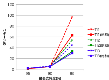
図 6 抽出数 (心不全)
