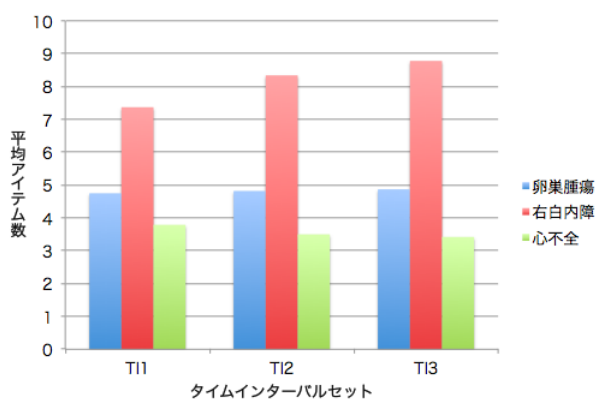
図 7 最低支持度 85%における頻出オーダ列の平均アイテム数
