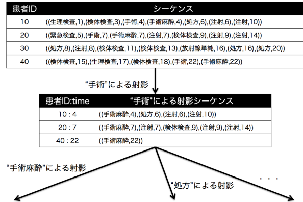
図 2 本手法のプレフィックススパンの流れ
