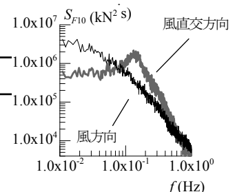
図2 頂部層風力のパワースペクトル密度
